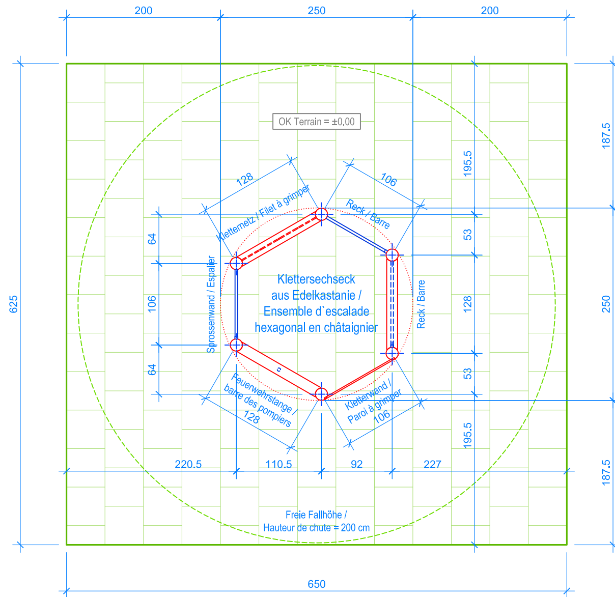
GRUNDRISS / PLAN 1:50
