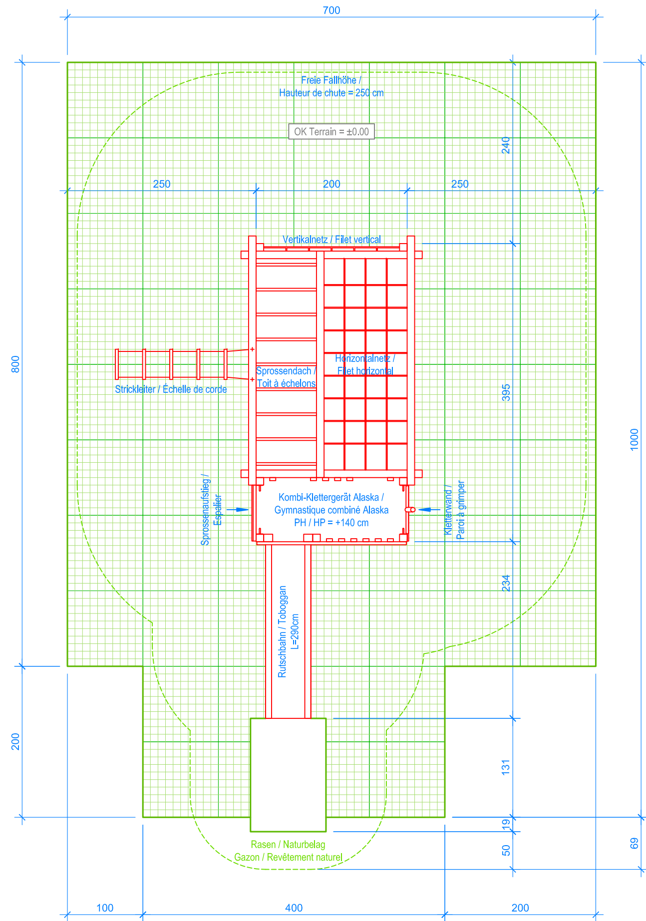
GRUNDRISS / PLAN 1:50
