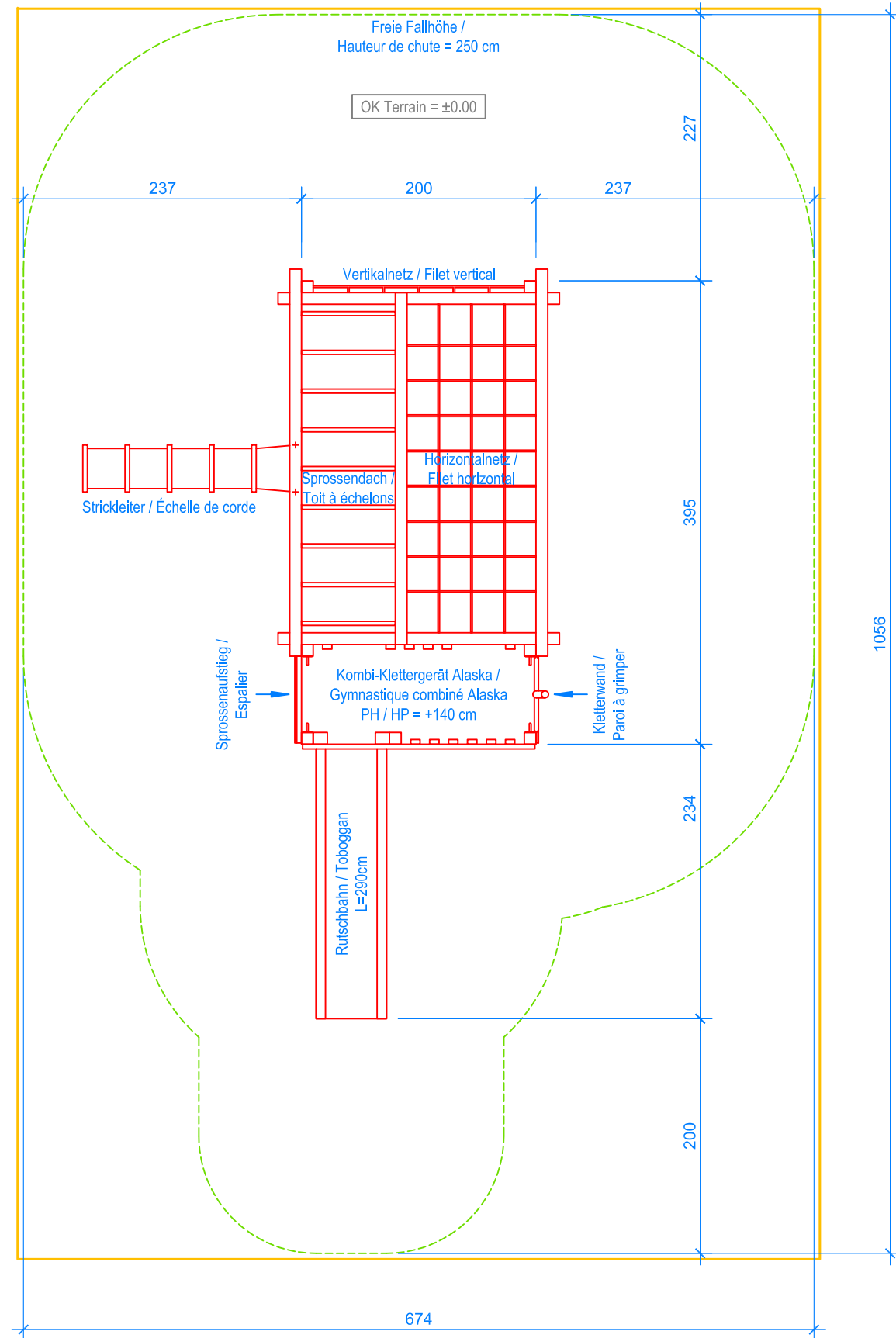
GRUNDRISS / PLAN 1:50
