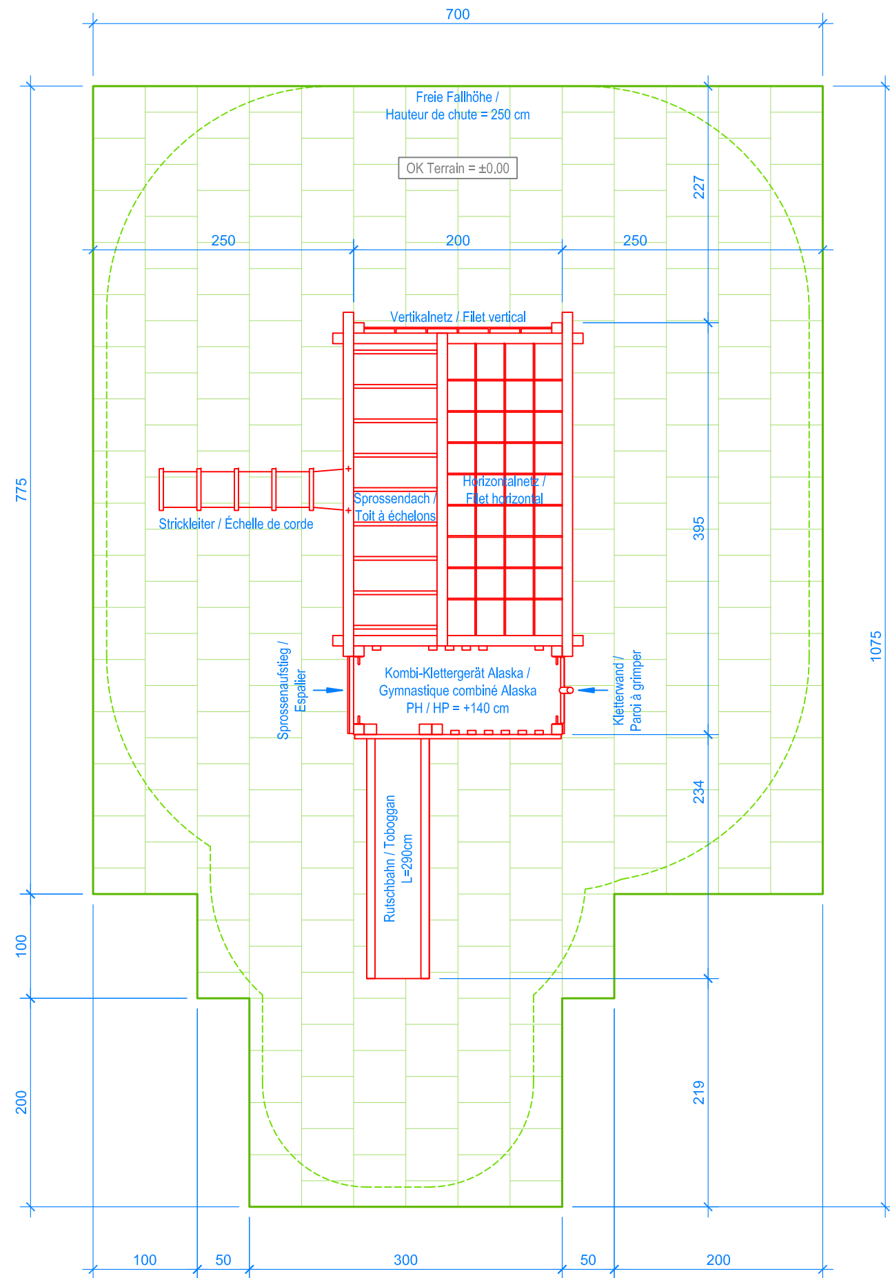
GRUNDRISS / PLAN 1:50
