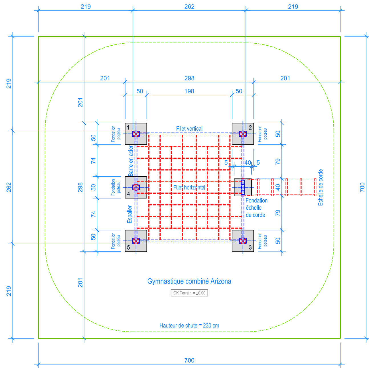
PLAN 1:50
