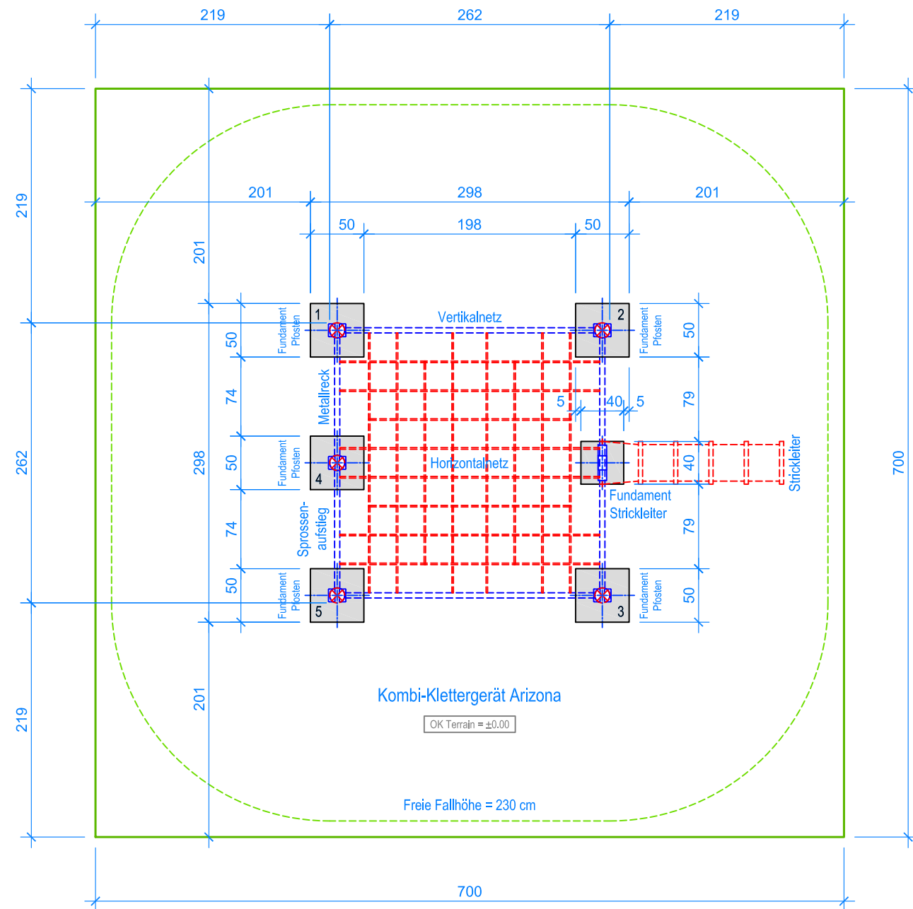
GRUNDRISS 1:50
