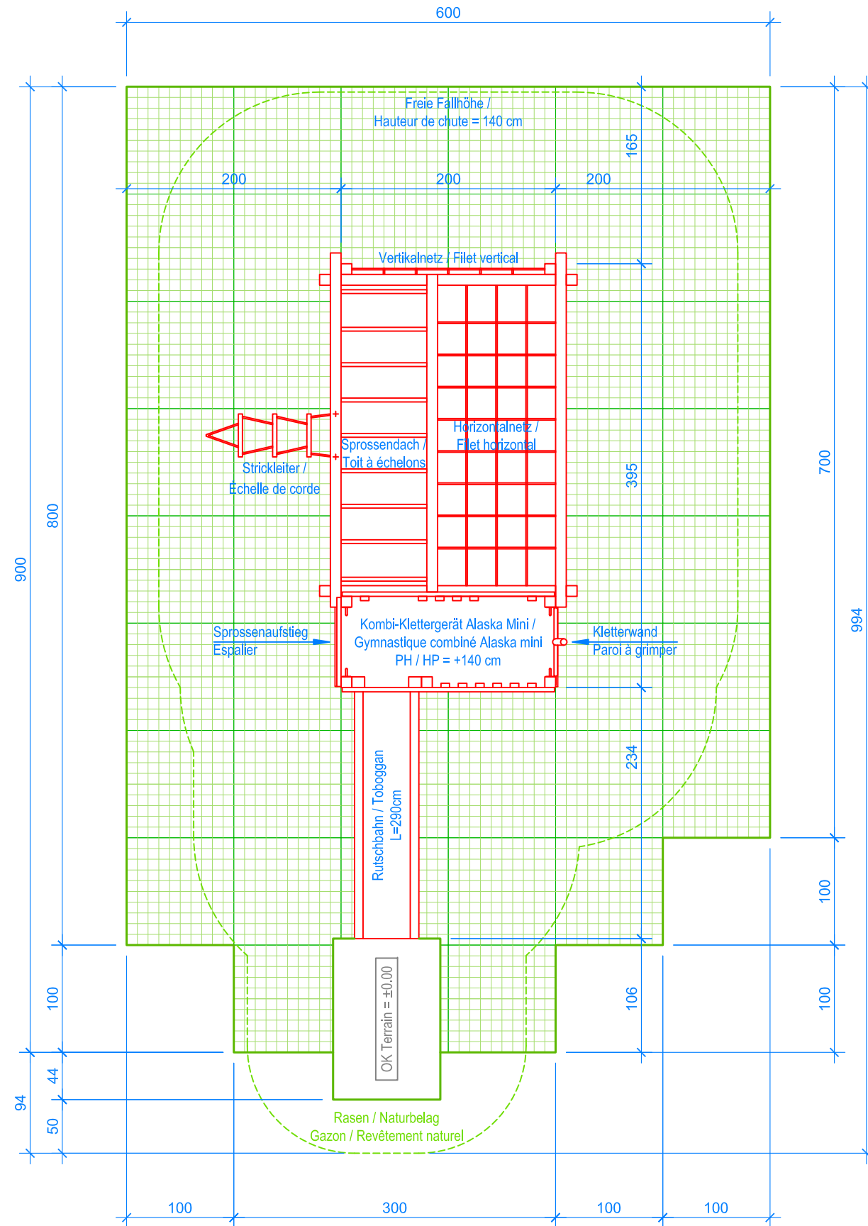
GRUNDRISS / PLAN 1:50
