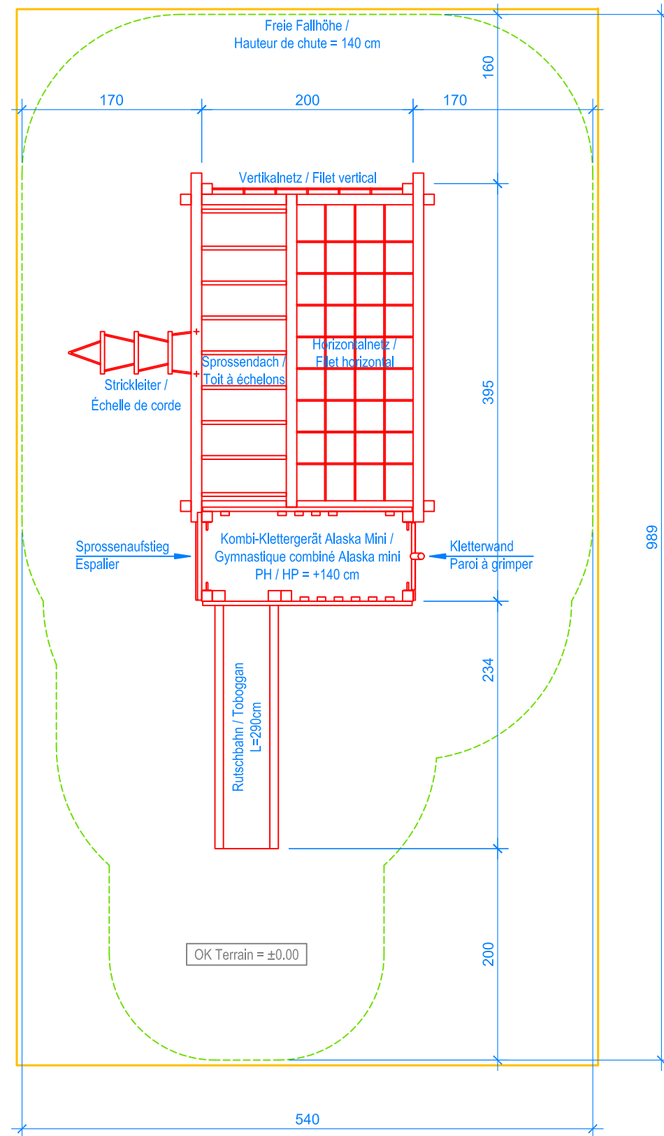
GRUNDRISS / PLAN 1:50
