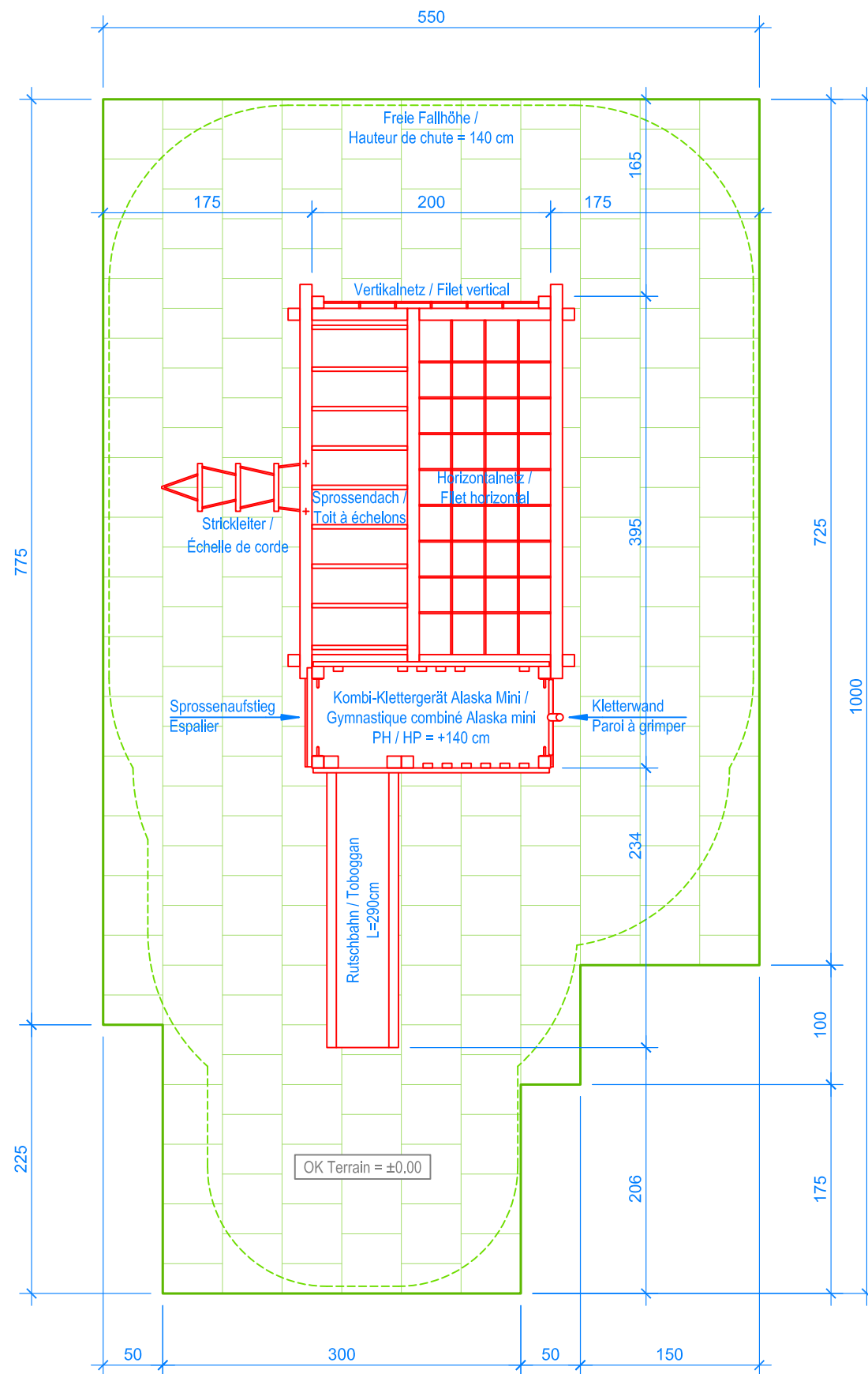
GRUNDRISS / PLAN 1:50
