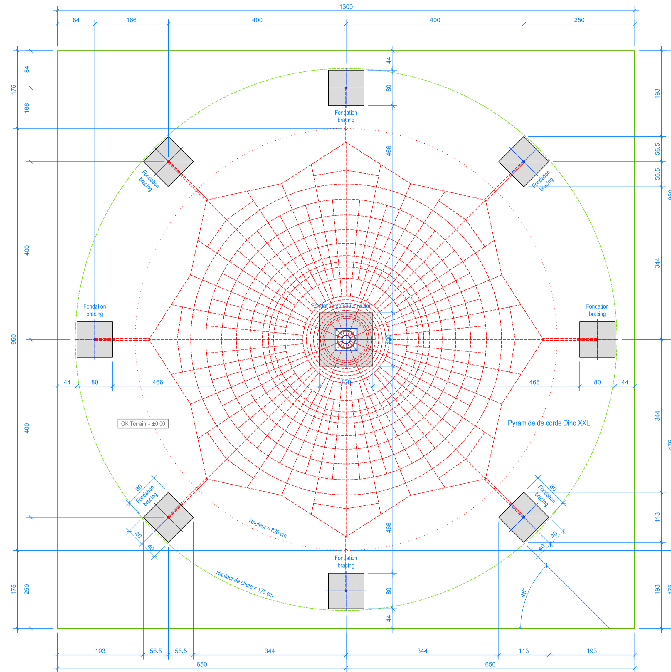
PLAN 1:50
