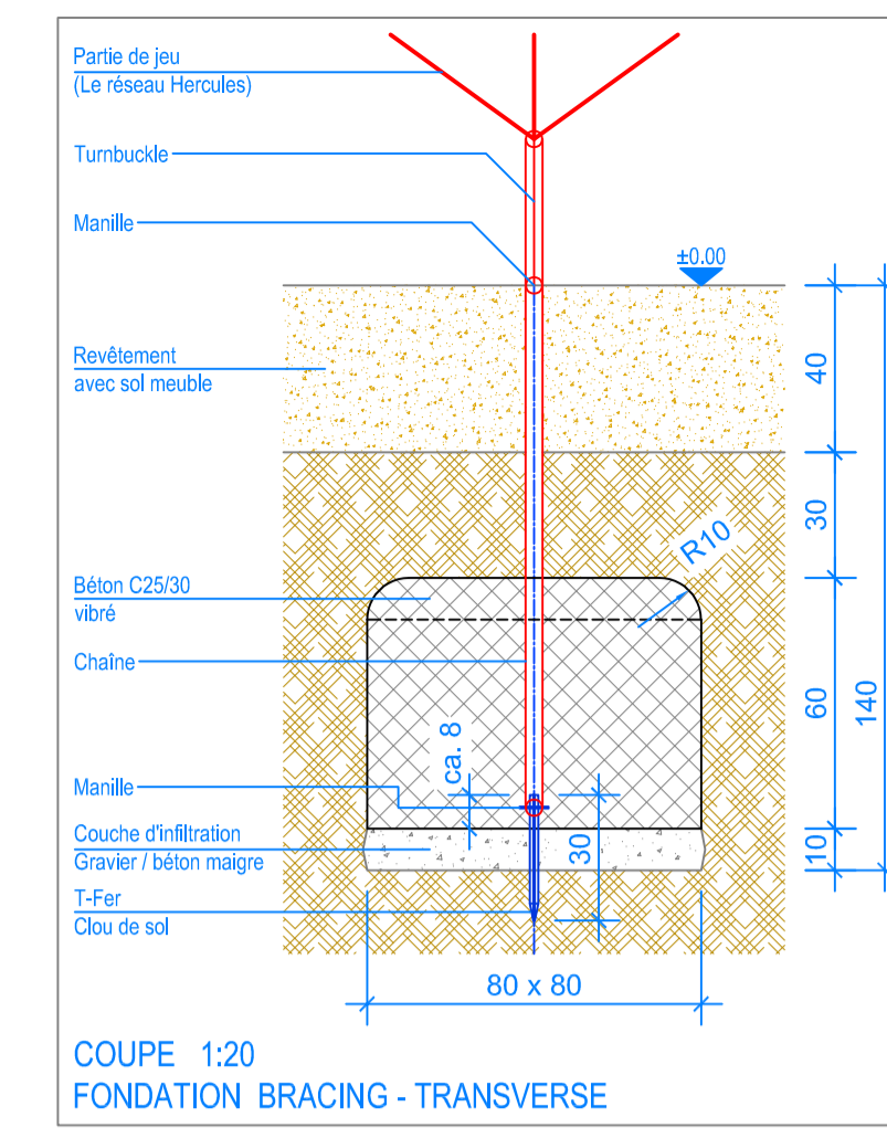
COUPE 1:20 FONDATION BRACING - TRANSVERSE
