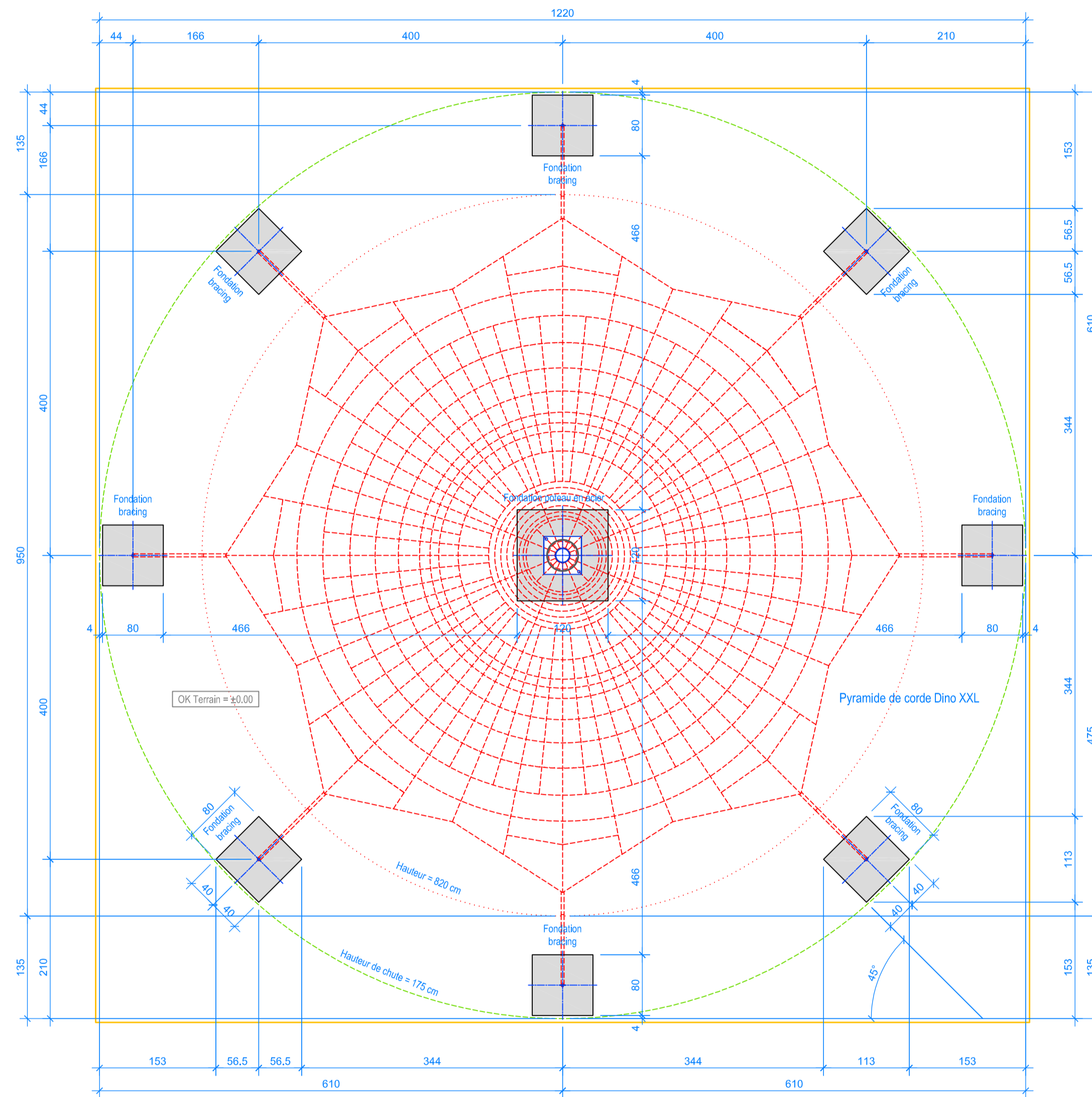
PLAN 1:50
