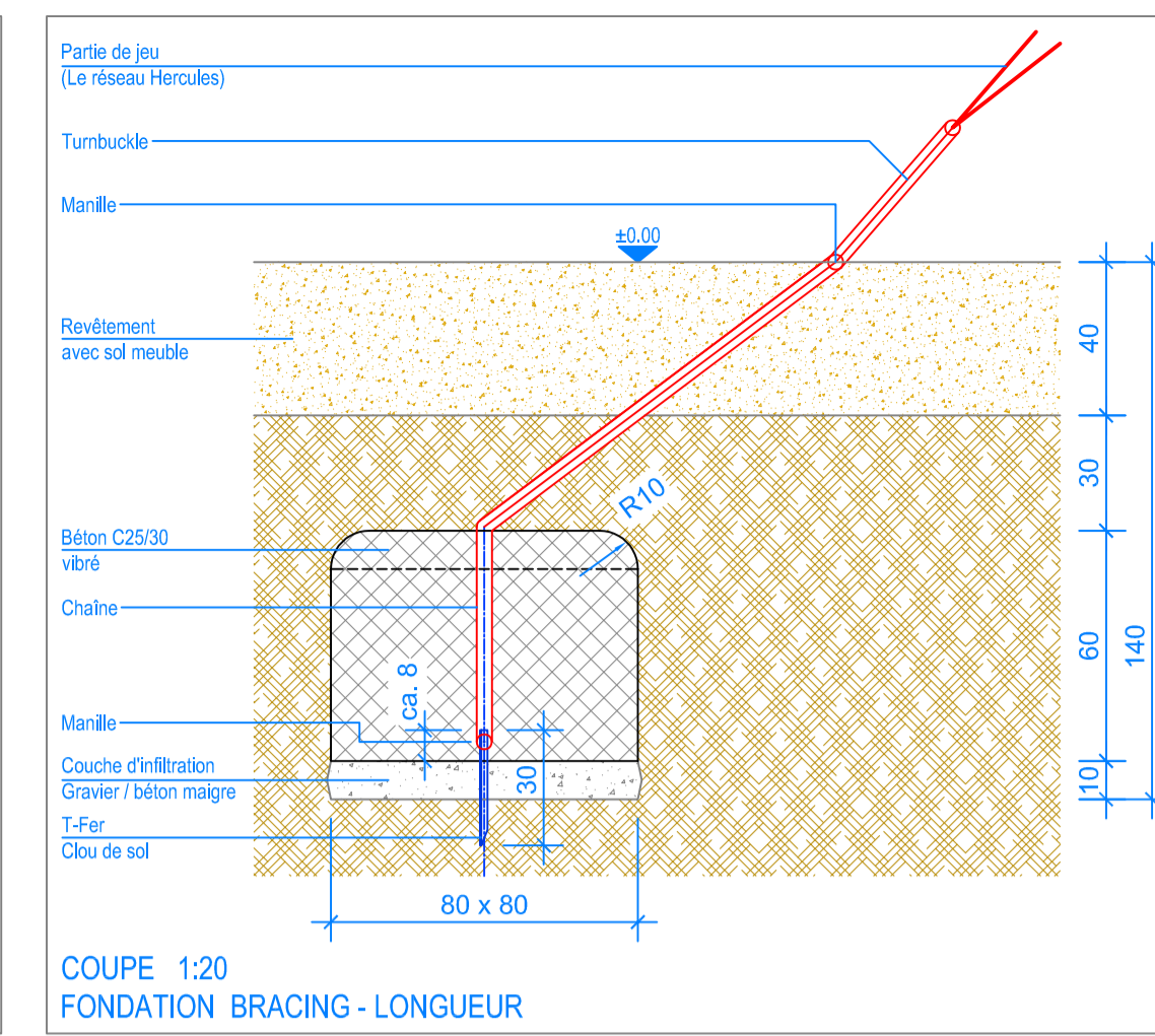
COUPE 1:20 FONDATION BRACING - LONGUEUR
