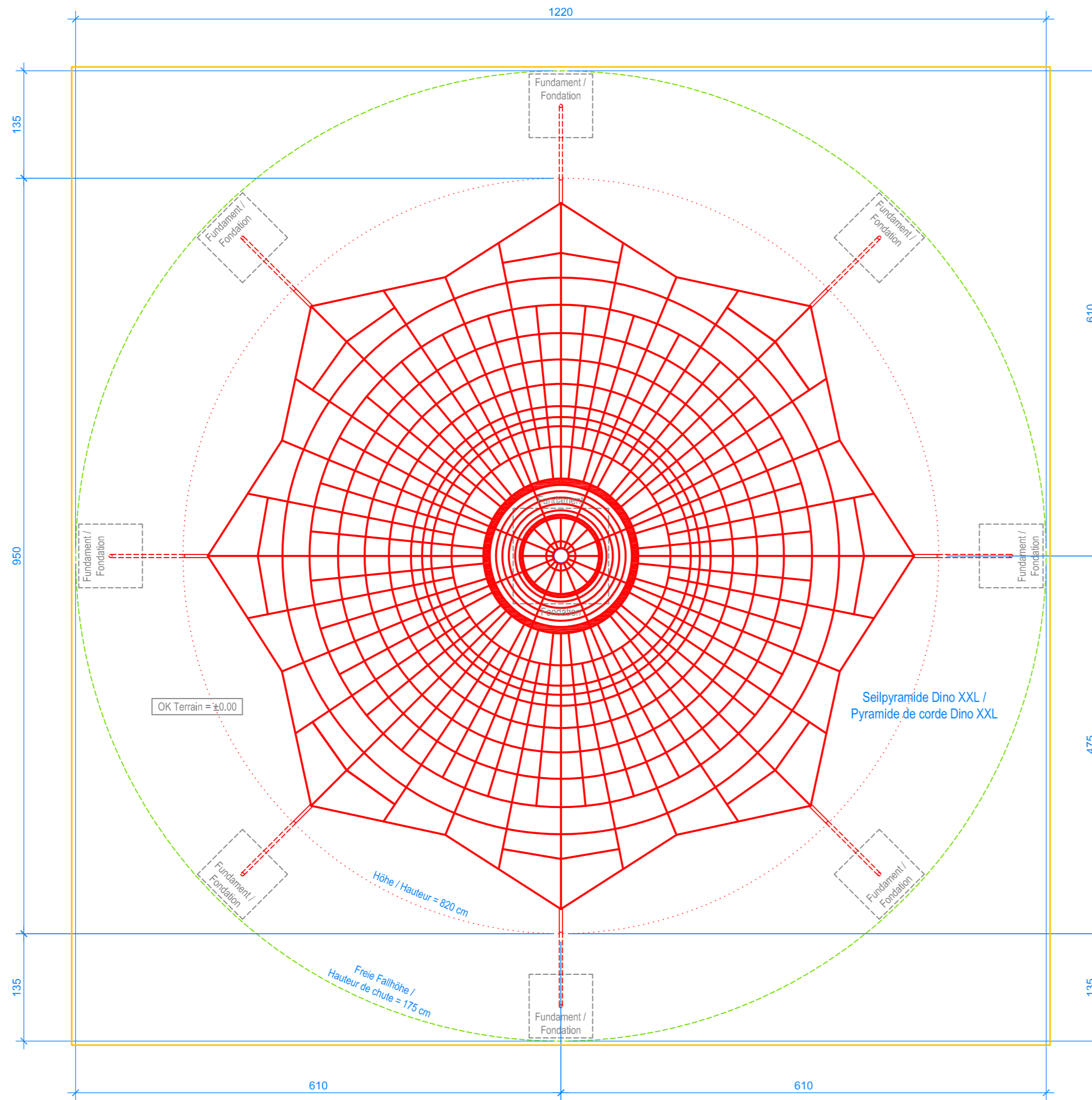
GRUNDRISS / PLAN 1:50
