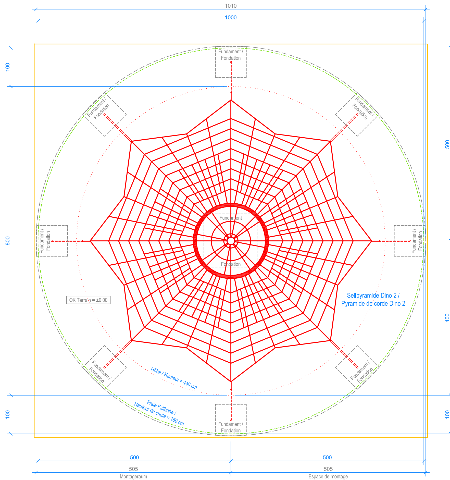
GRUNDRISS / PLAN 1:50
