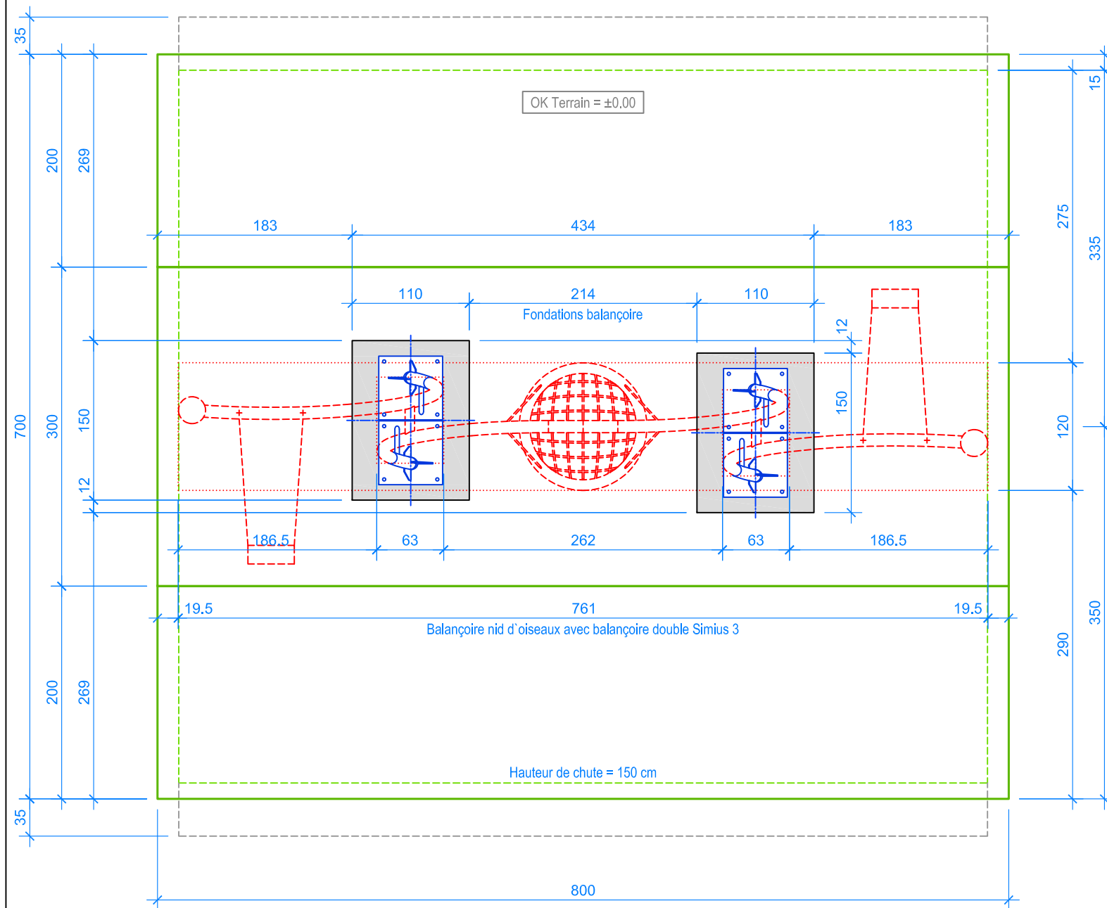
PLAN 1:50
