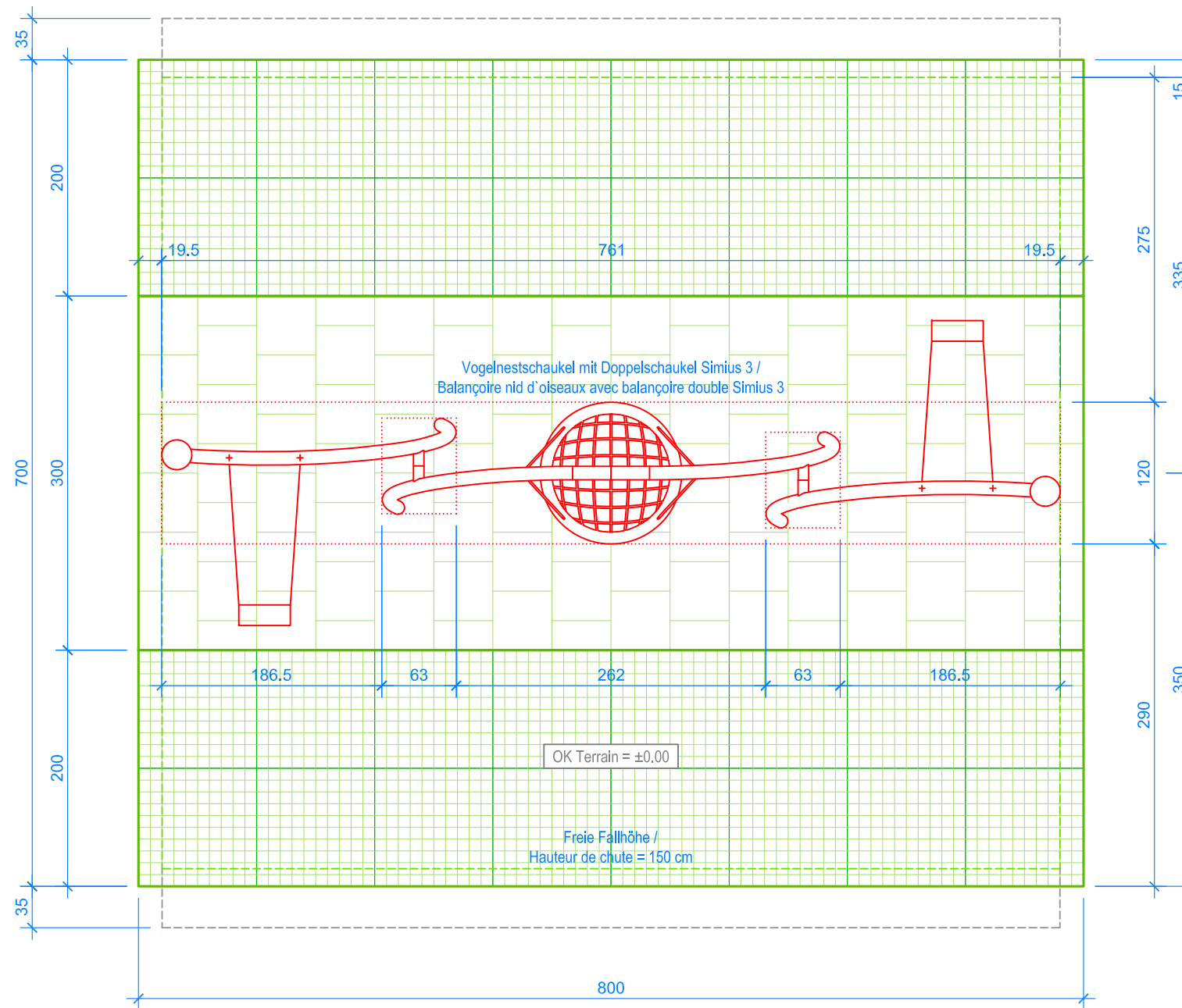
GRUNDRISS / PLAN 1:50
