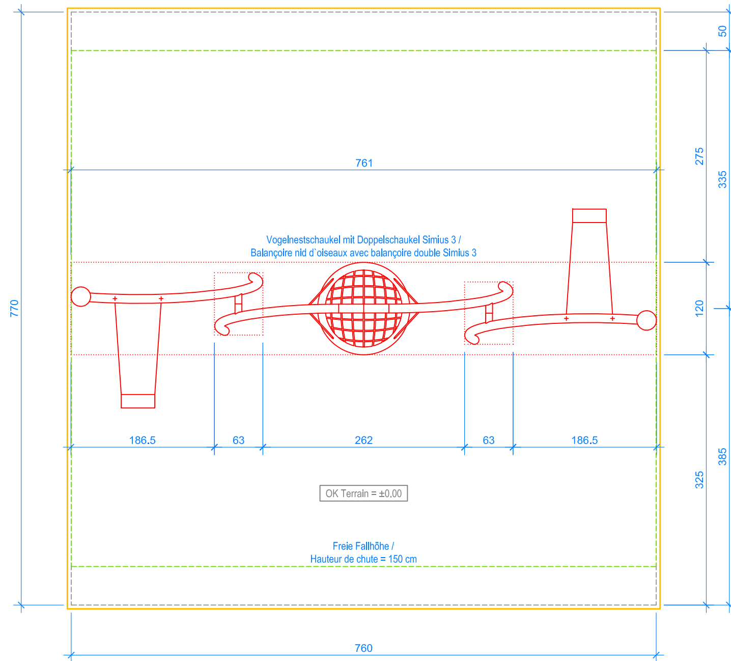
GRUNDRISS / PLAN 1:50
