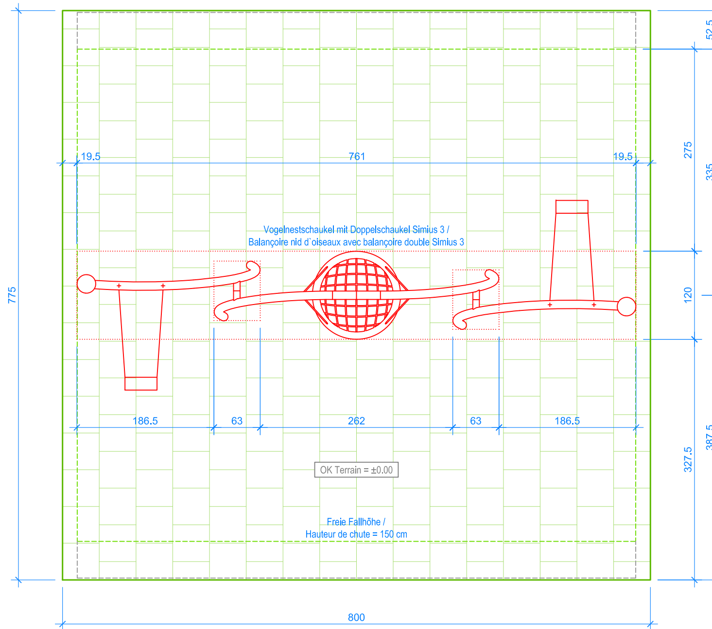
GRUNDRISS / PLAN 1:50
