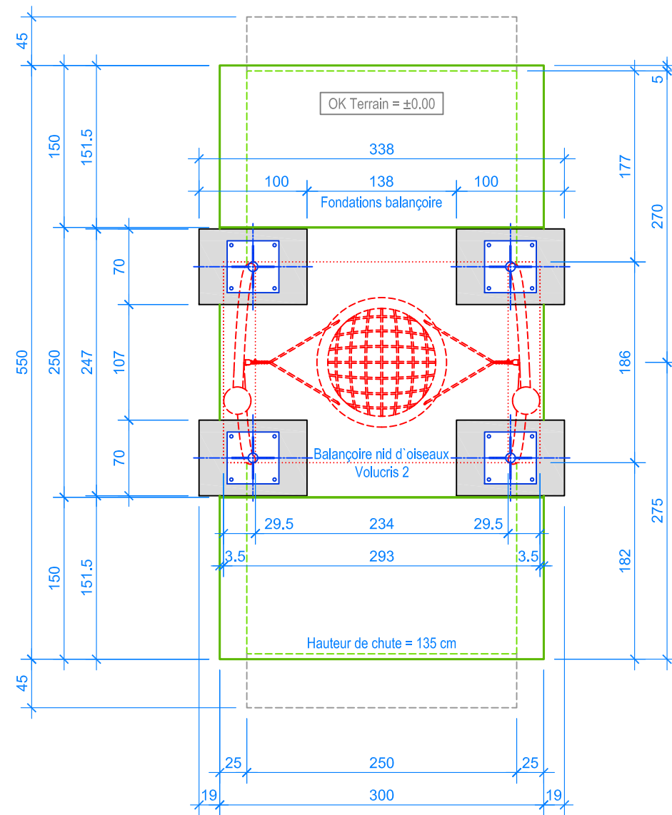
PLAN 1:50
