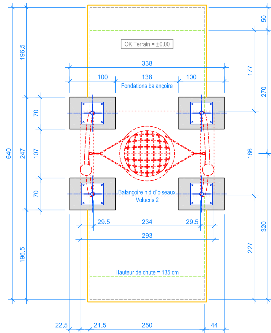
PLAN 1:50
