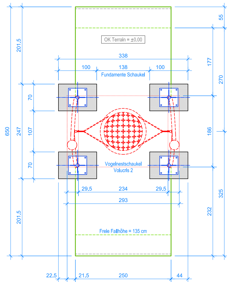
GRUNDRISS 1:50
