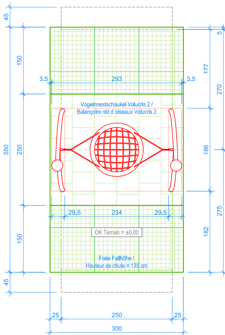
GRUNDRISS / PLAN 1:50
