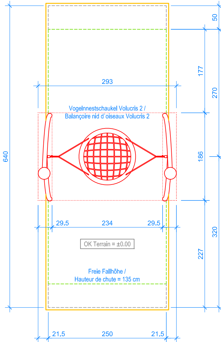
GRUNDRISS / PLAN 1:50
