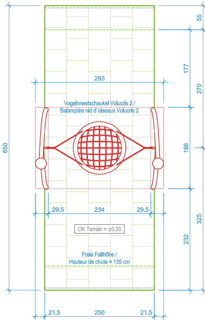
GRUNDRISS / PLAN 1:50
