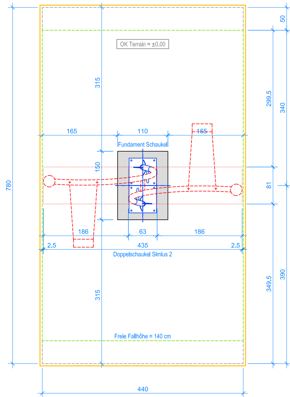
GRUNDRISS 1:50
