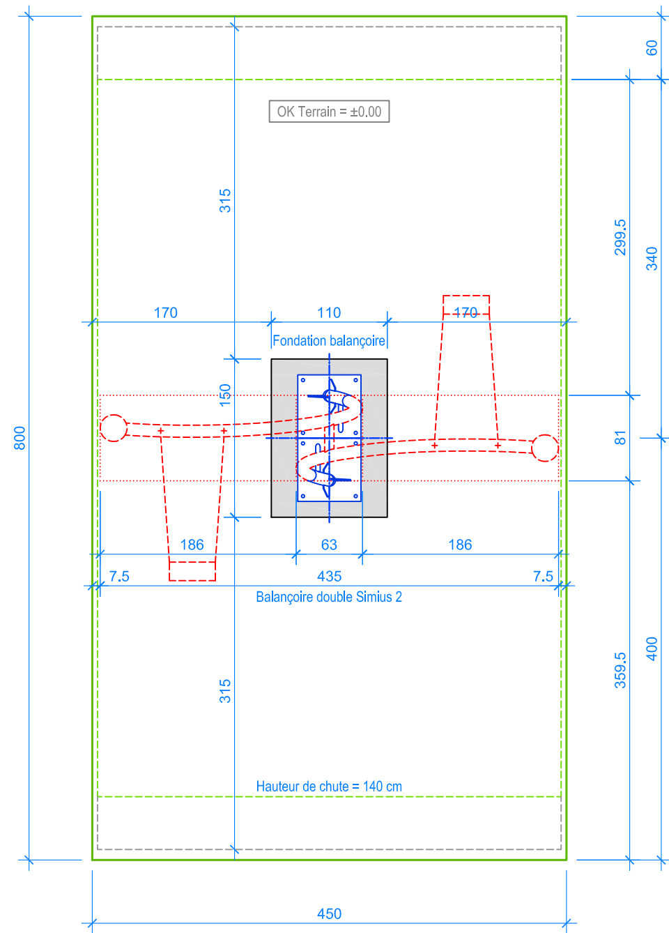
PLAN 1:50
