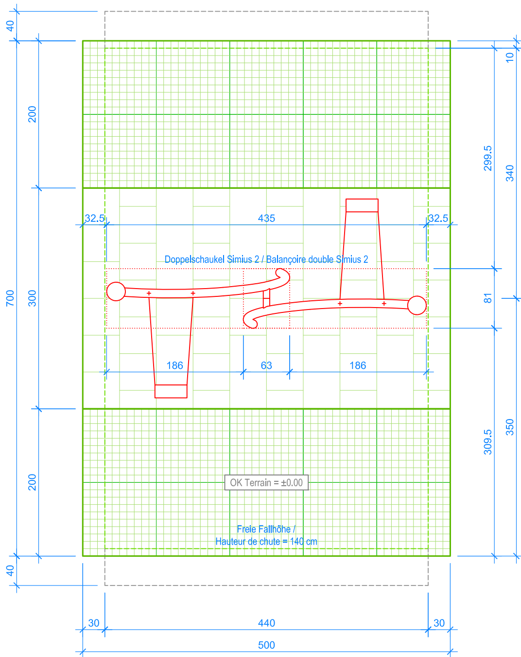
GRUNDRISS / PLAN 1:50
