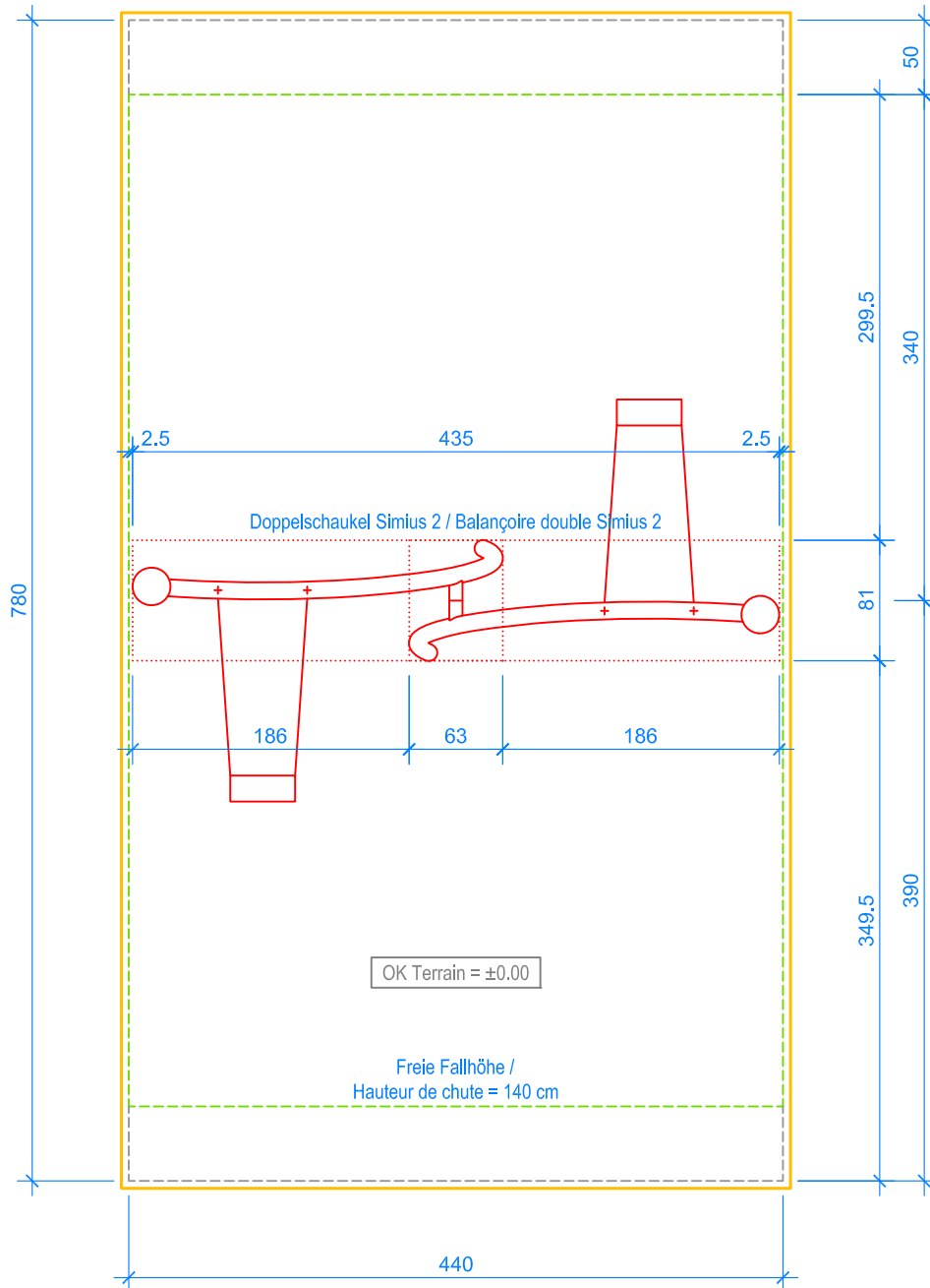
GRUNDRISS / PLAN 1:50
