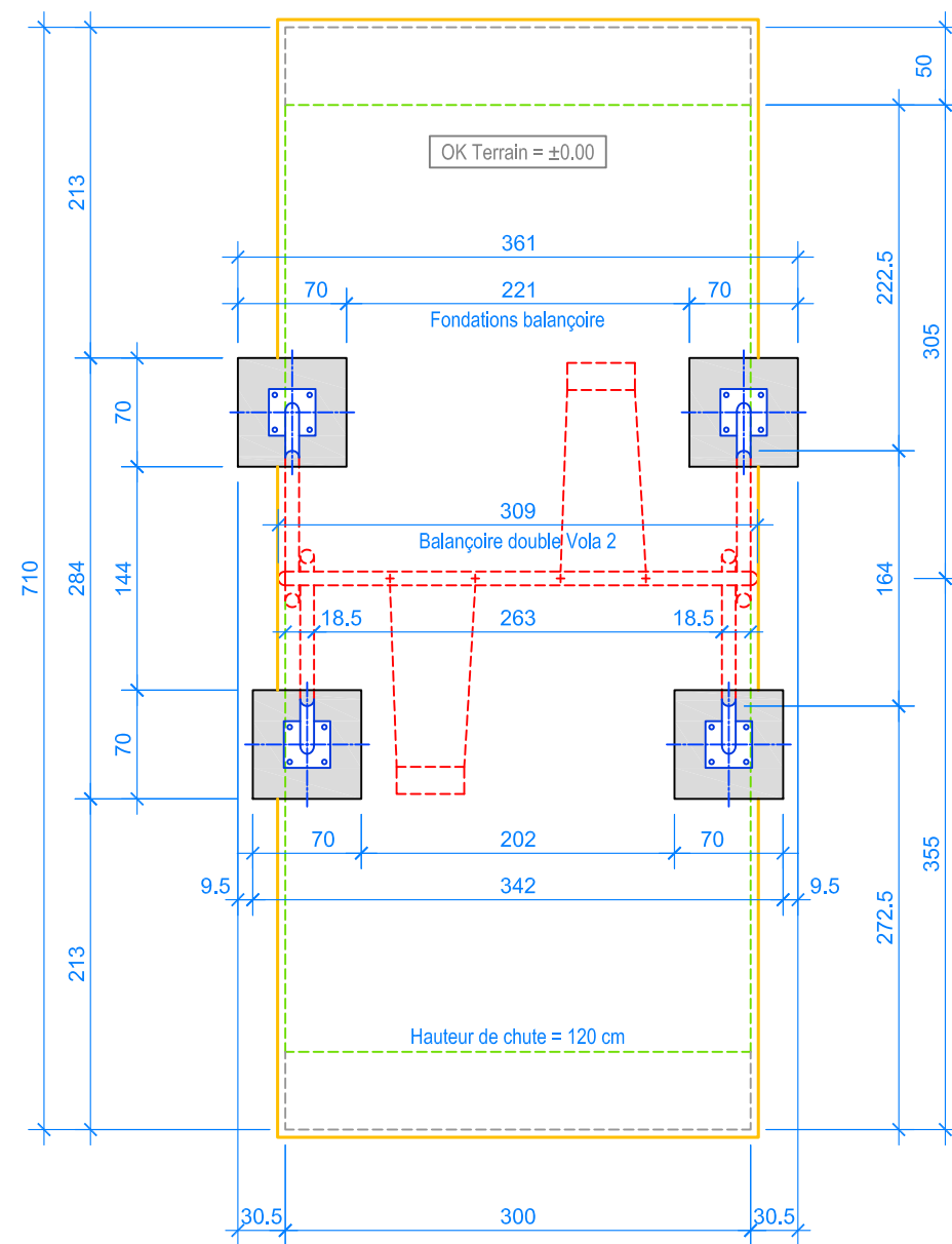
PLAN 1:50
