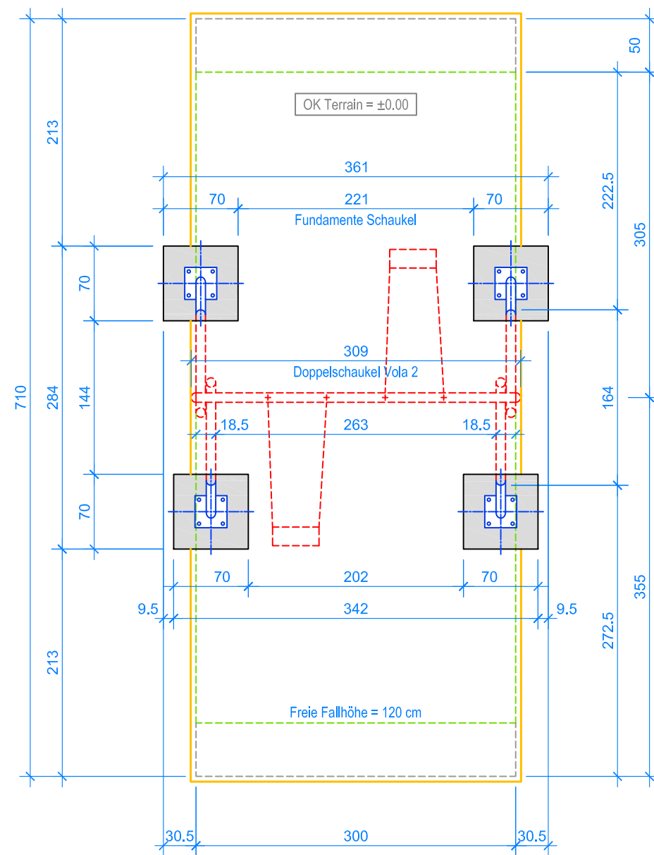
GRUNDRISS 1:50
