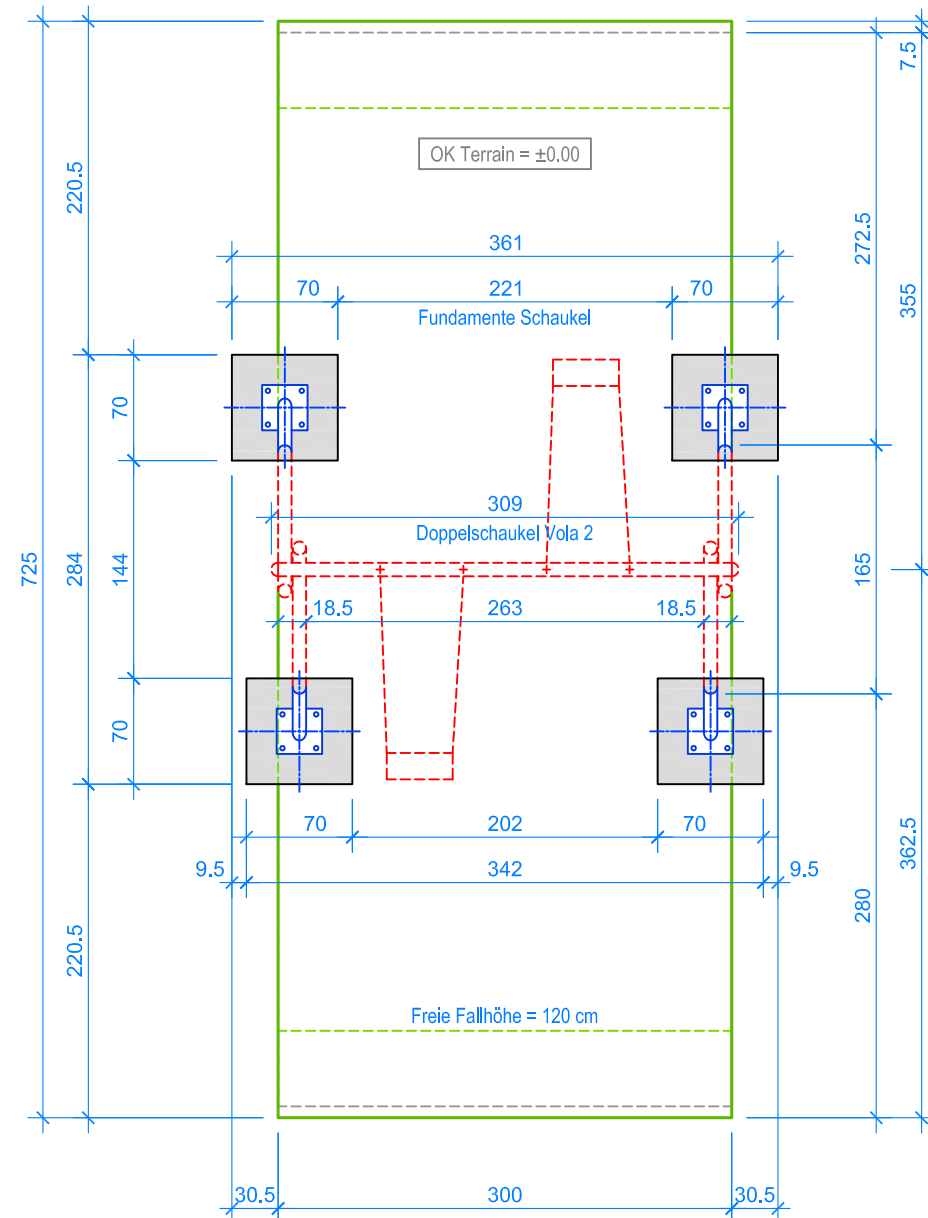
GRUNDRISS 1:50
