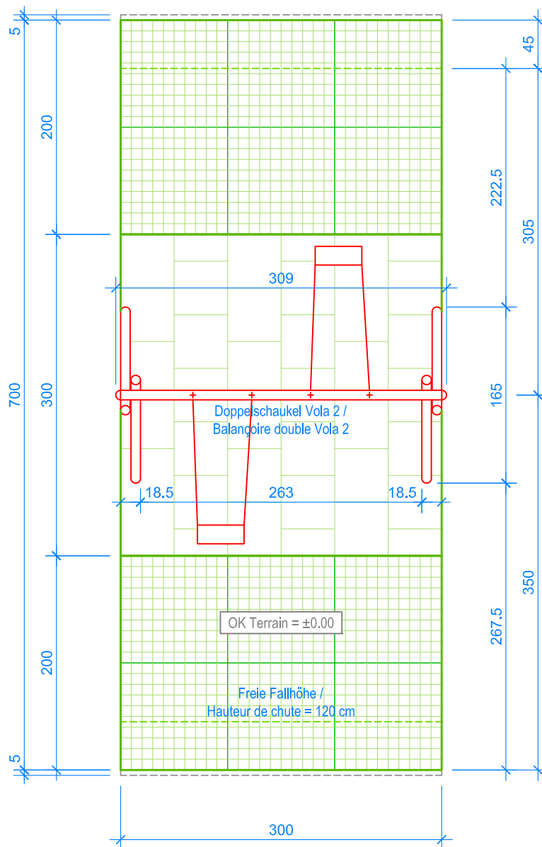
GRUNDRISS / PLAN 1:50
