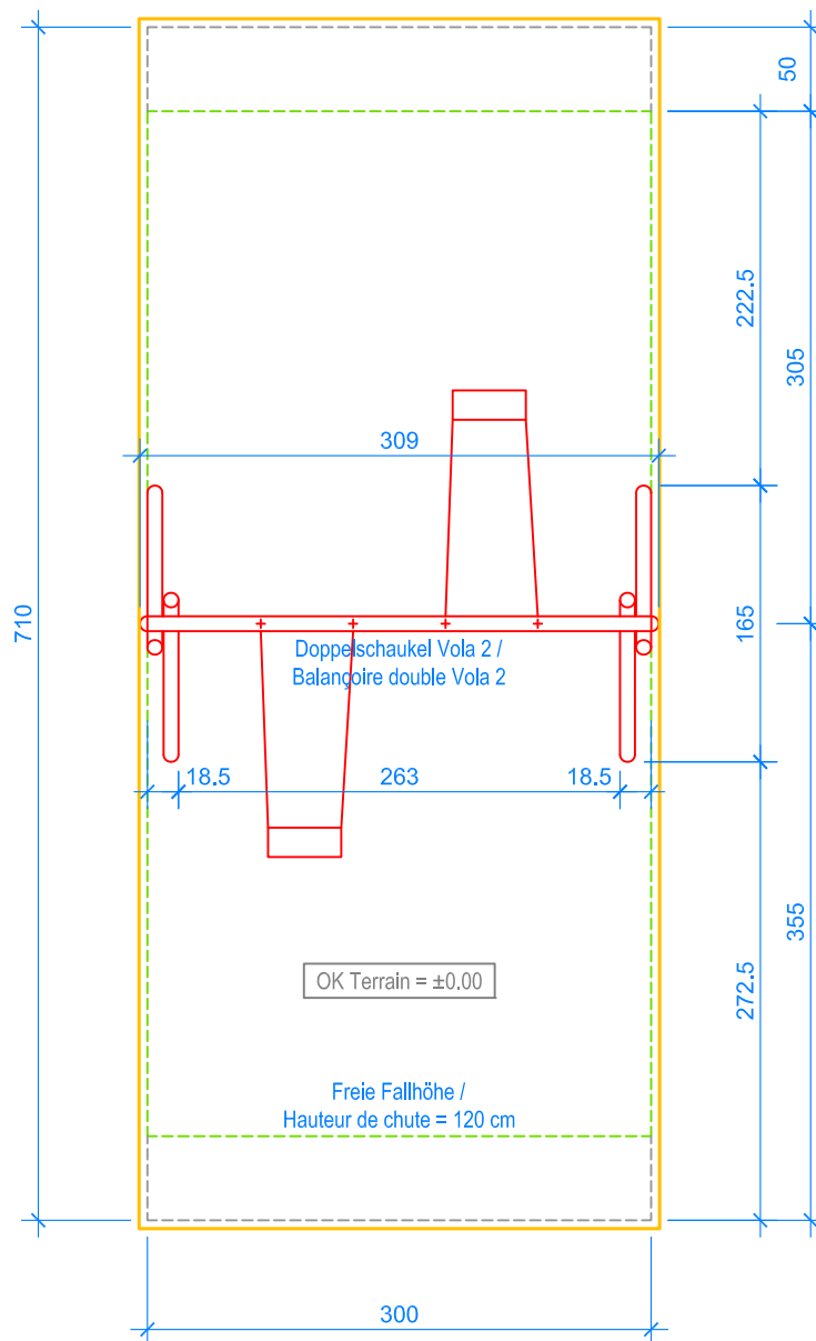
GRUNDRISS / PLAN 1:50
