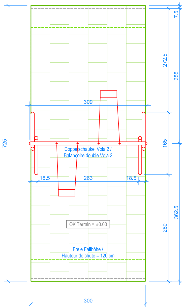
GRUNDRISS / PLAN 1:50
