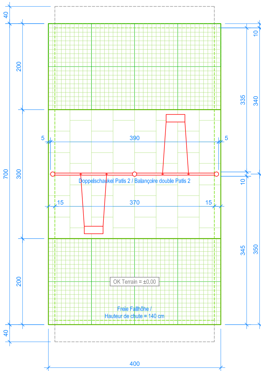
GRUNDRISS / PLAN 1:50
