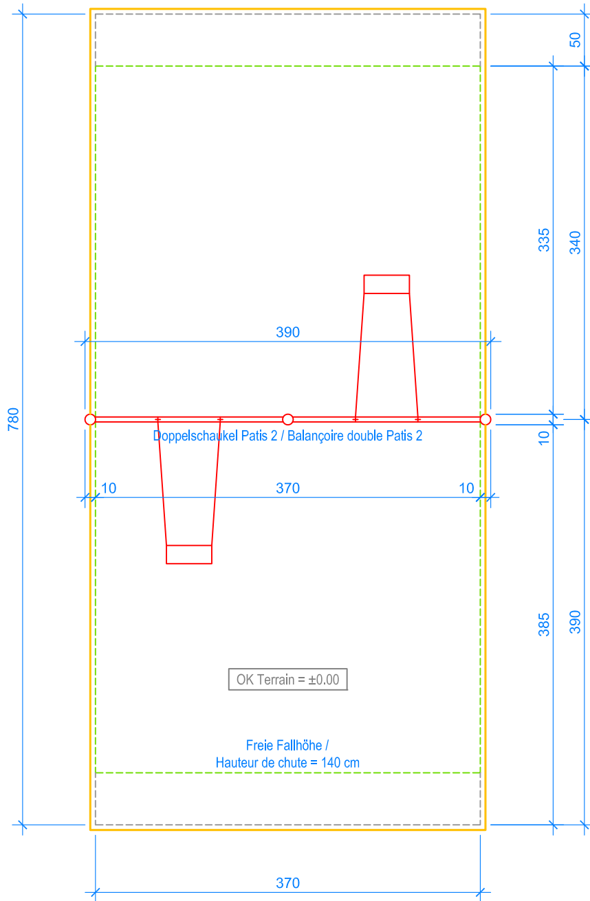
GRUNDRISS / PLAN 1:50
