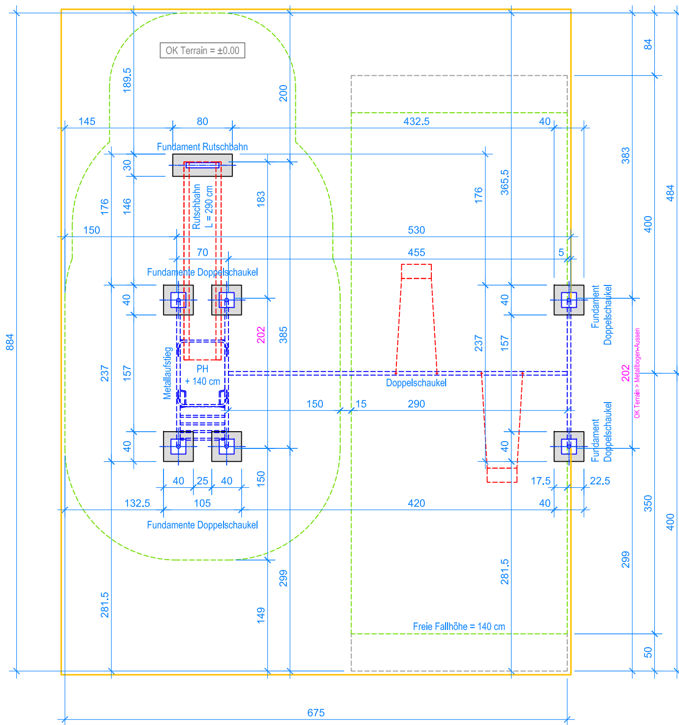
GRUNDRISS 1:50
