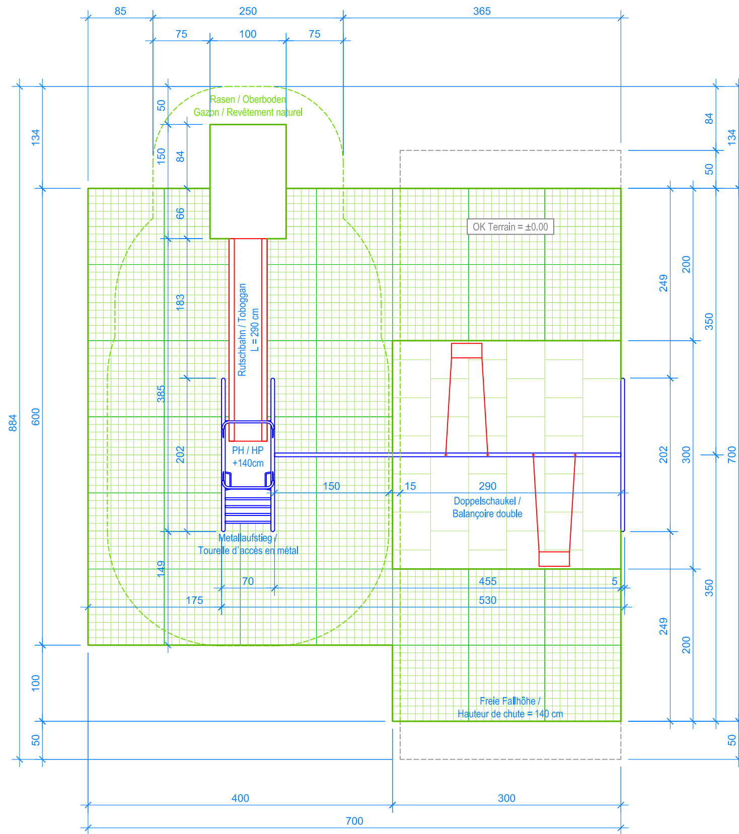
GRUNDRISS / PLAN 1:50
