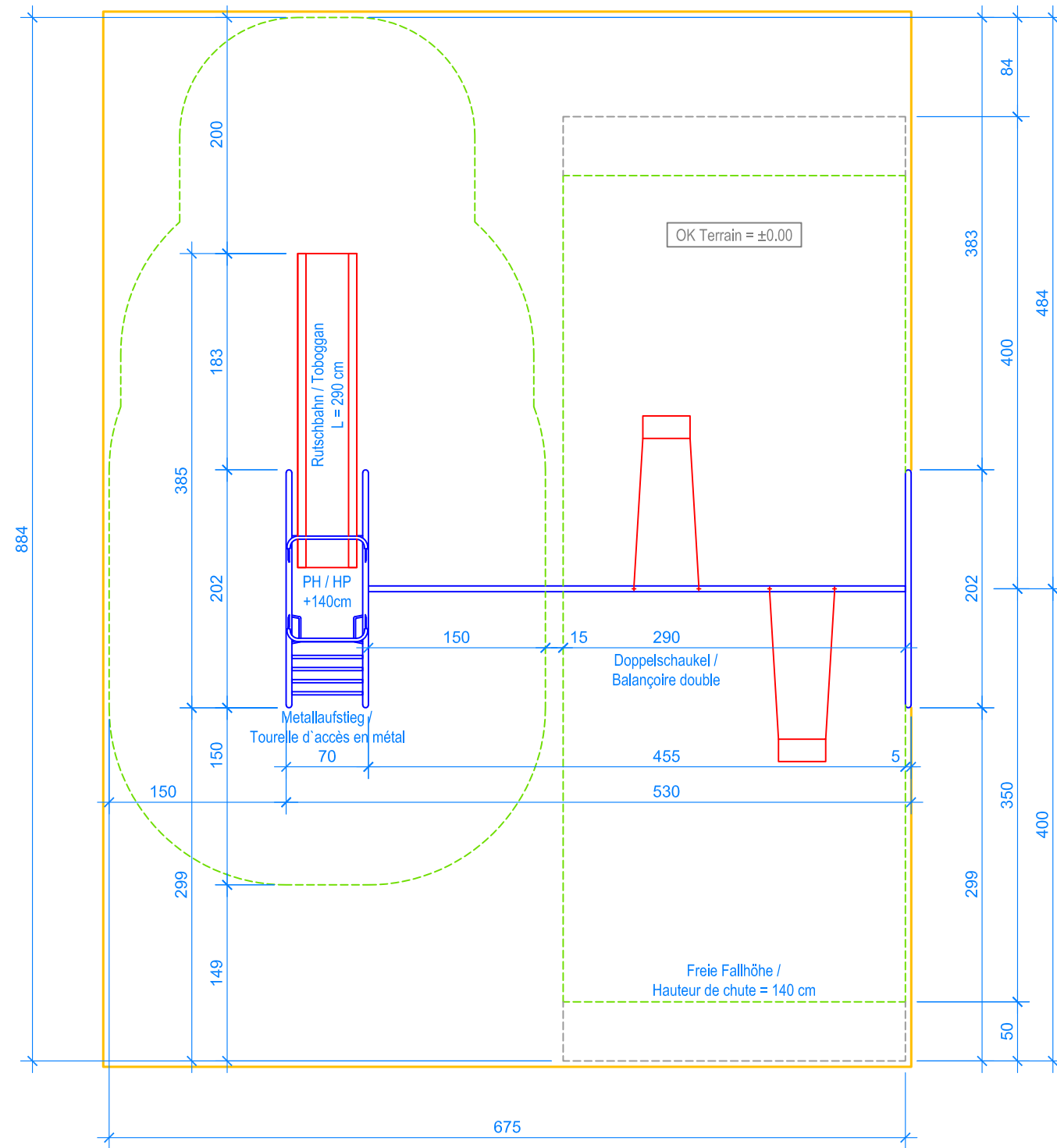
GRUNDRISS / PLAN 1:50
