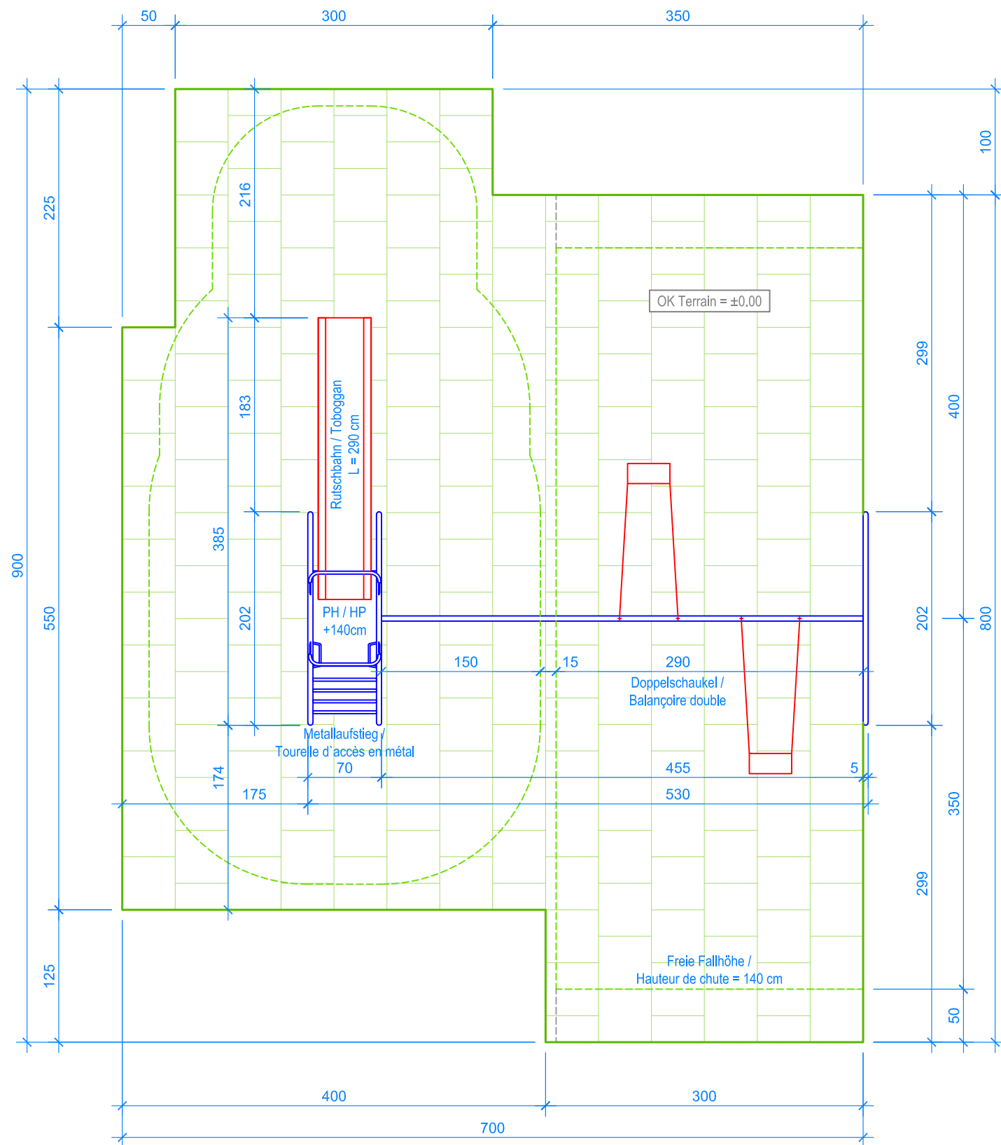
GRUNDRISS / PLAN 1:50
