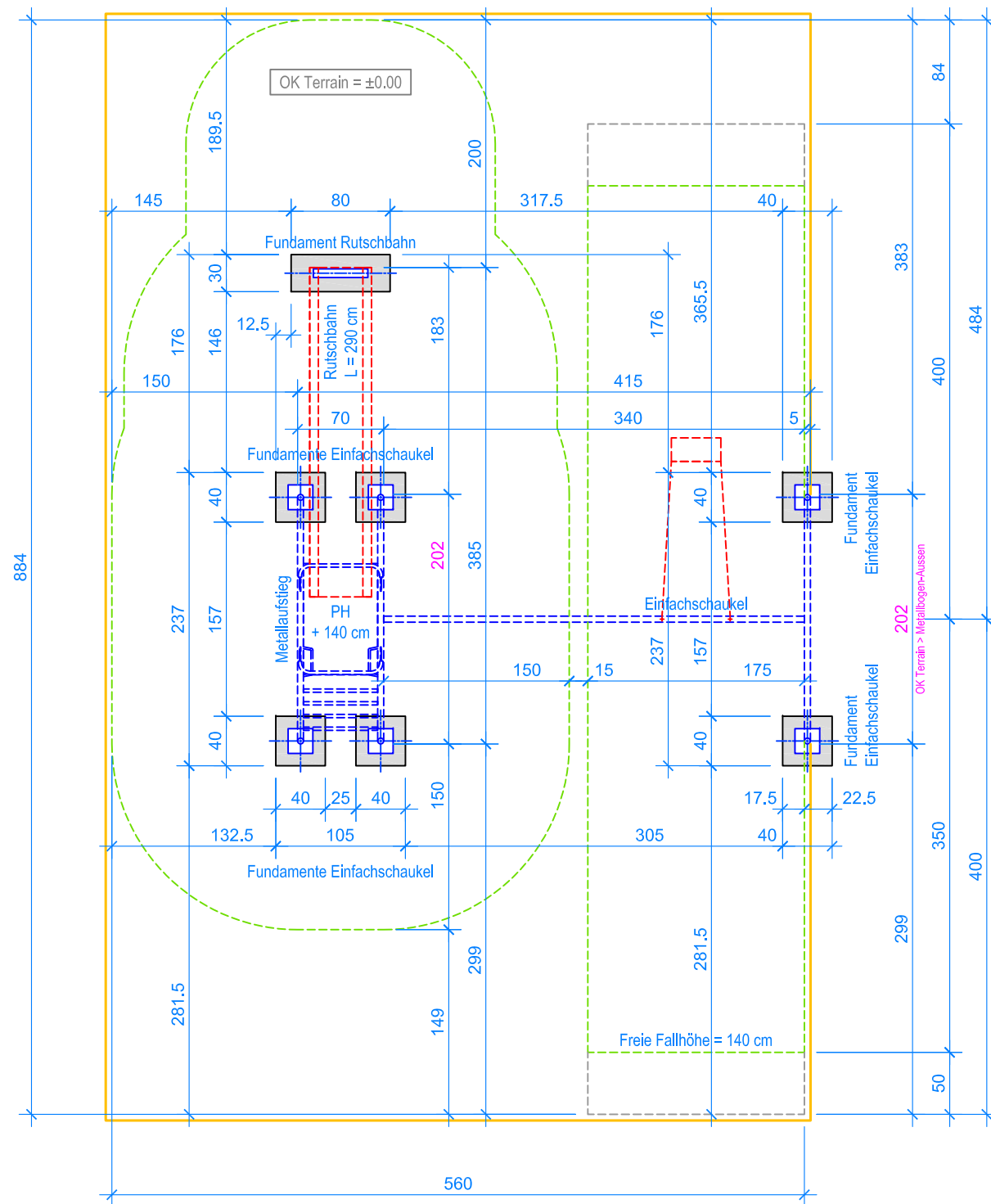
GRUNDRISS 1:50
