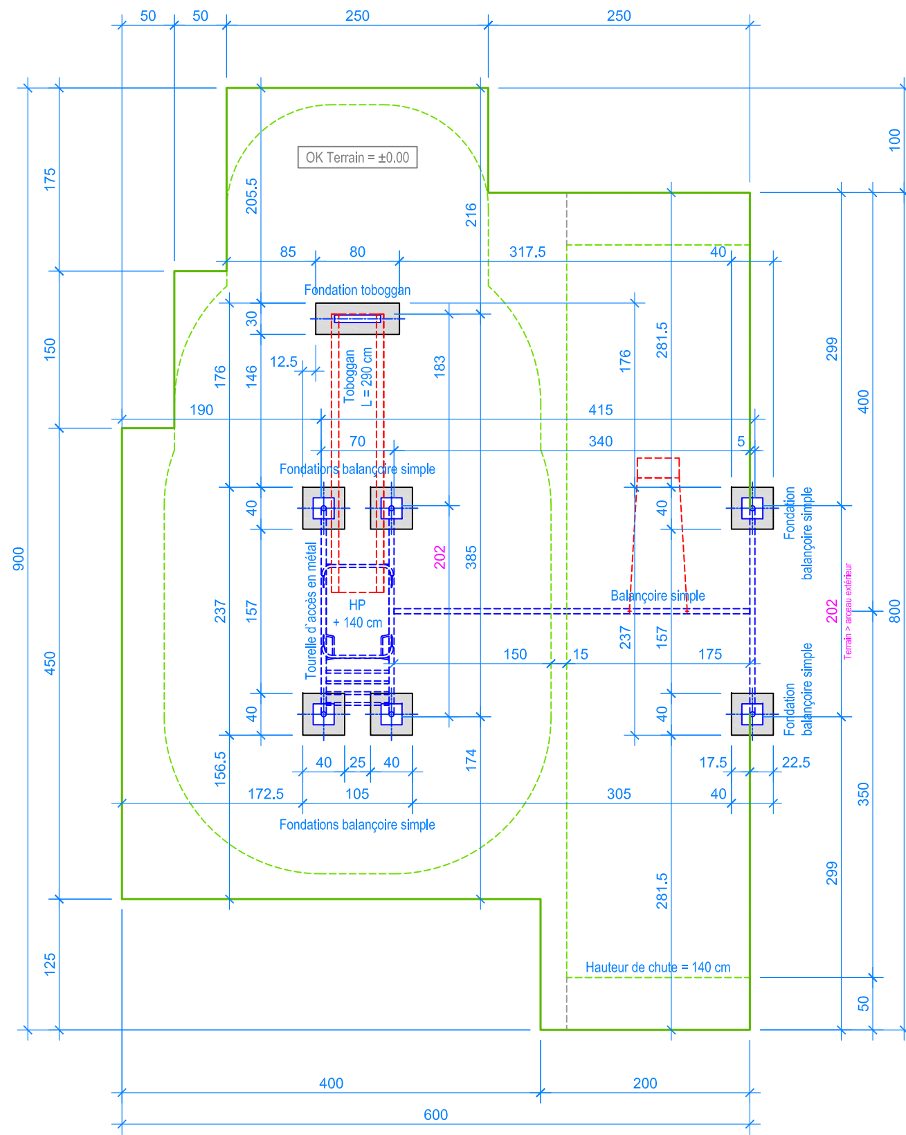
PLAN 1:50
