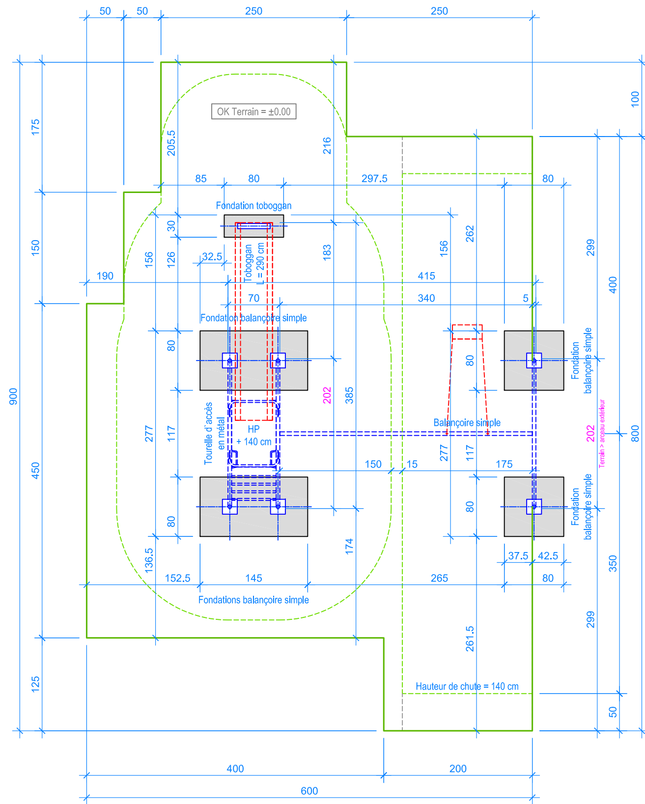
PLAN 1:50
