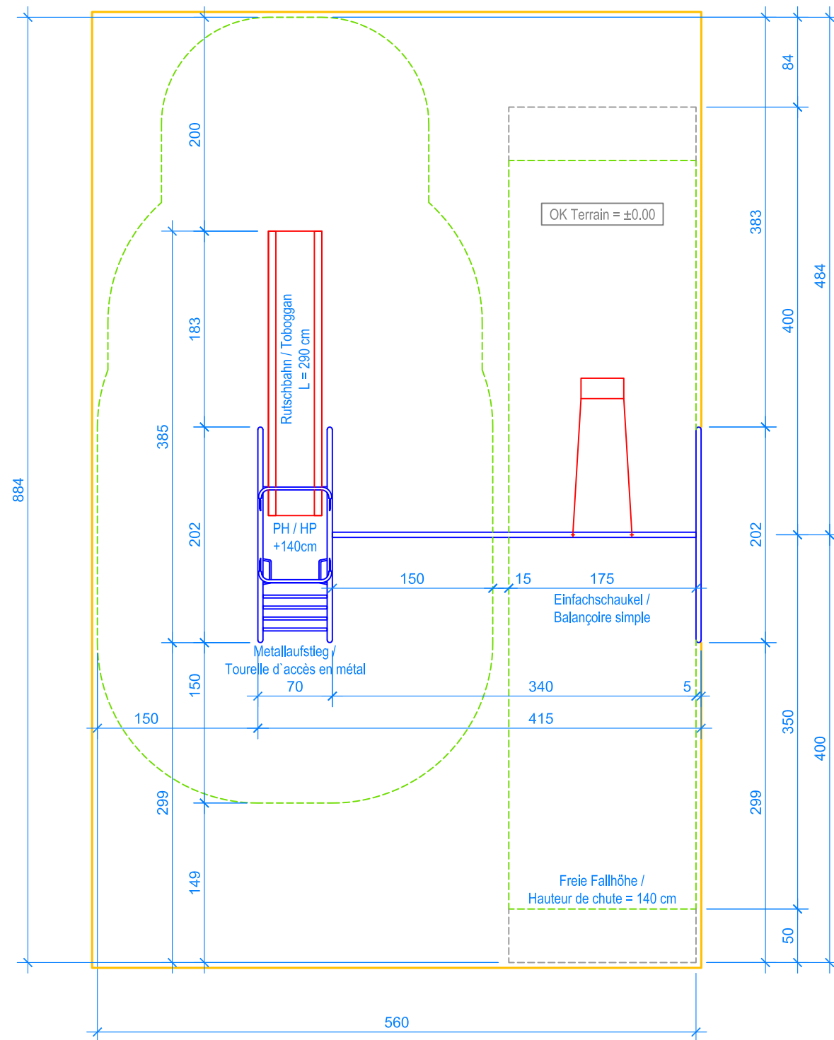
GRUNDRISS / PLAN 1:50
