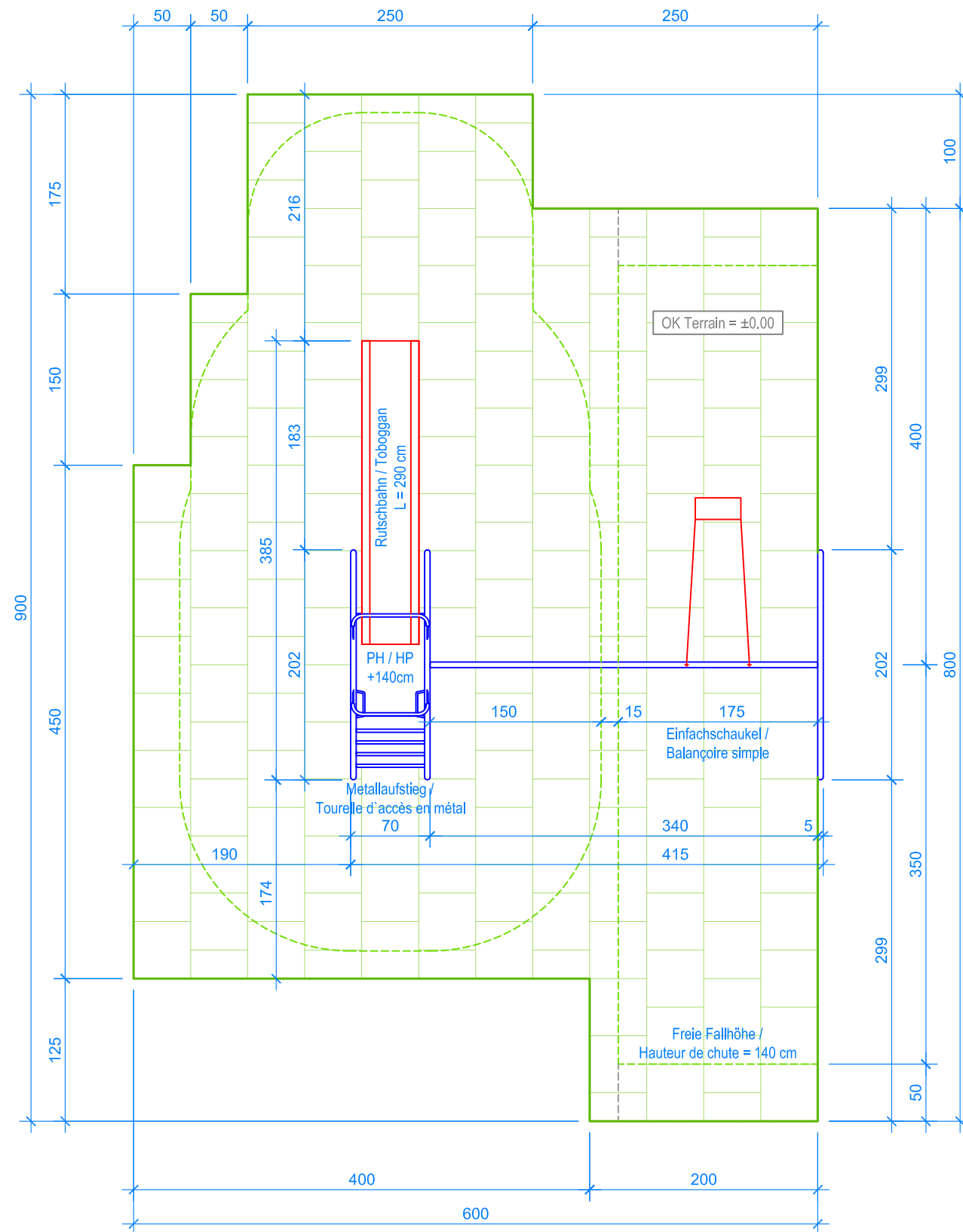
GRUNDRISS / PLAN 1:50
