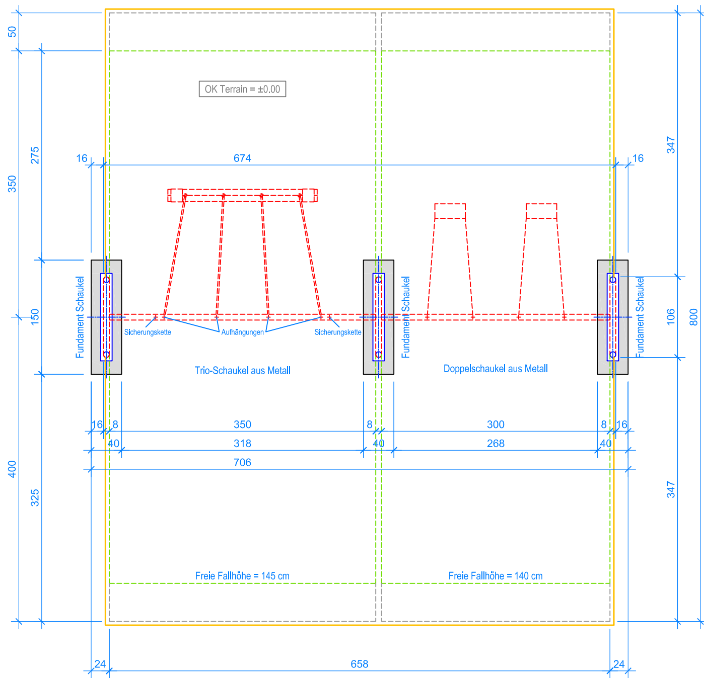
GRUNDRISS 1:50
