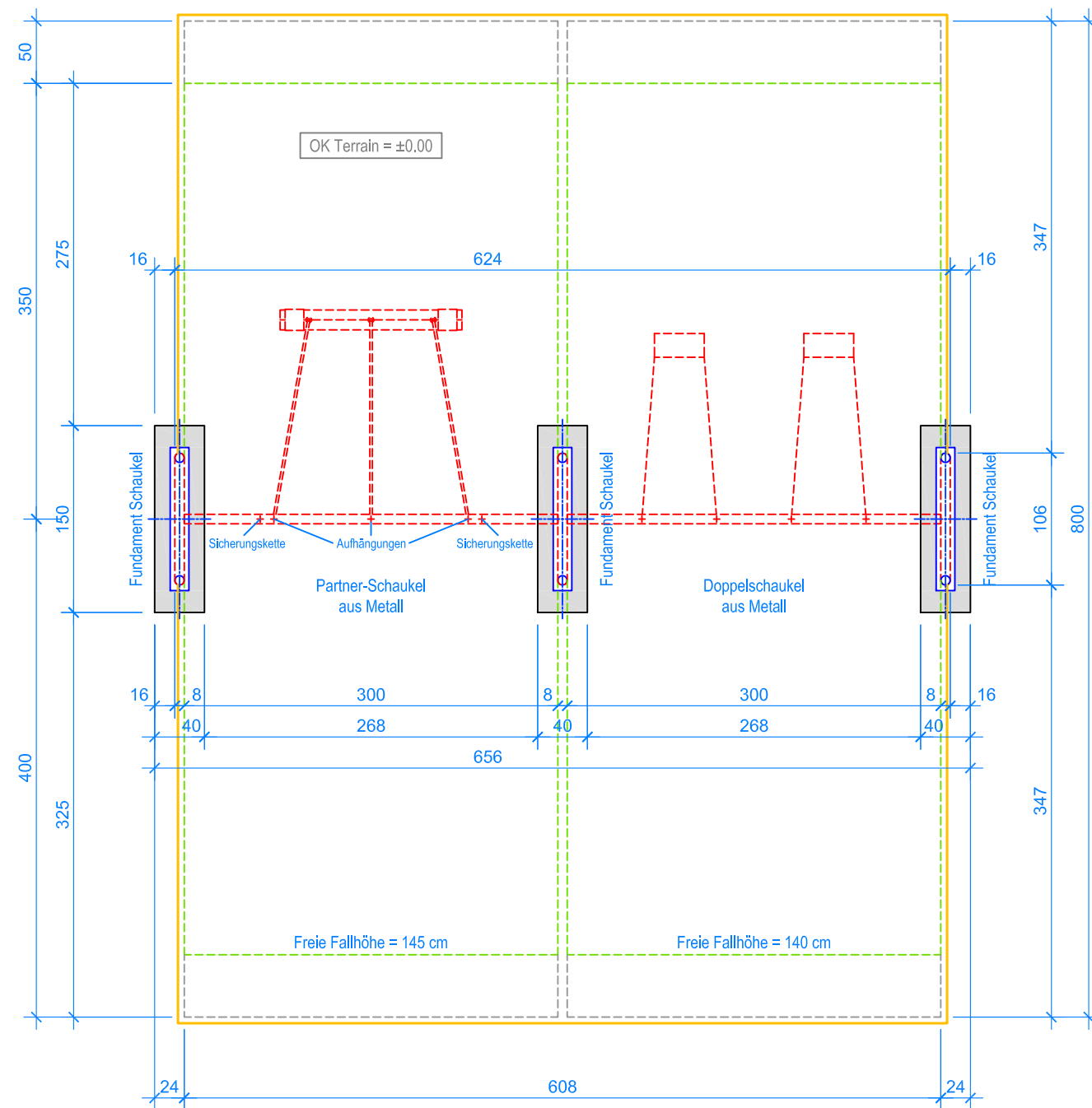
GRUNDRISS 1:50
