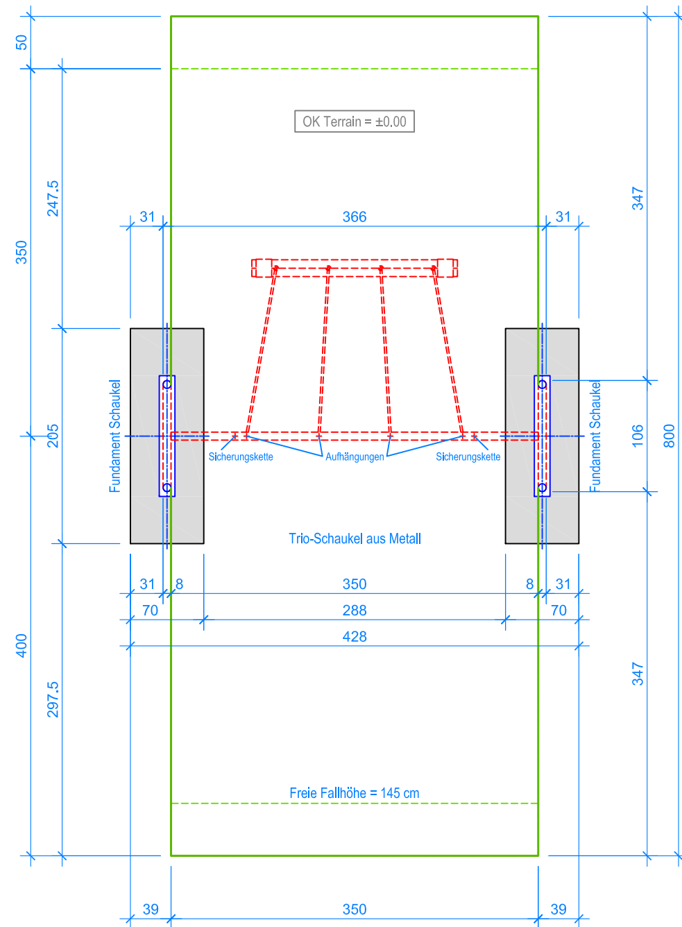
GRUNDRISS 1:50
