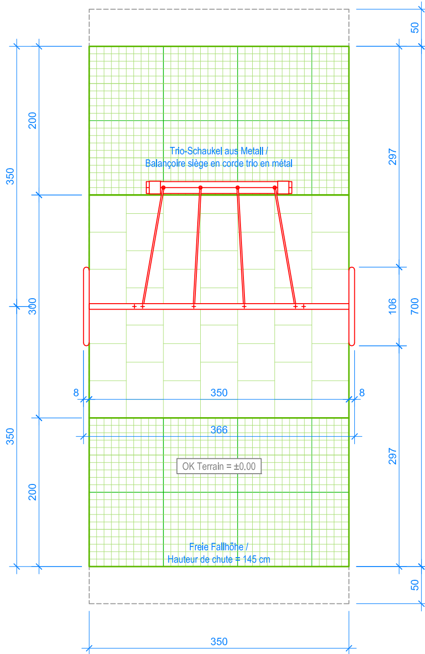
GRUNDRISS / PLAN 1:50
