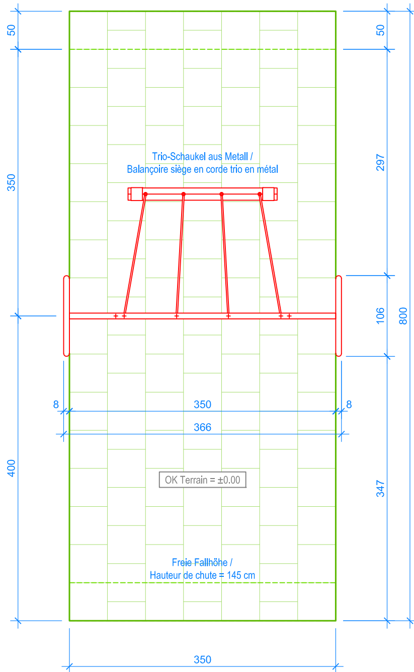
GRUNDRISS / PLAN 1:50
