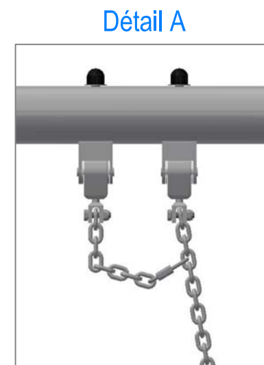
Chaîne de sécurité: Mousqueton à fixer dans le 4ème maillon
